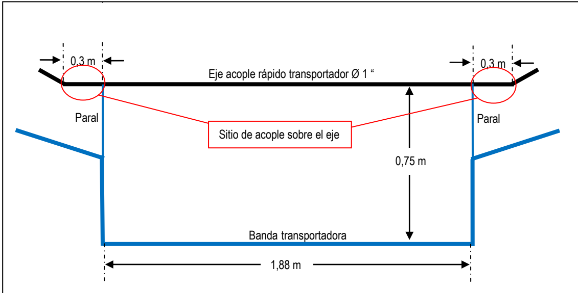
Fig. 1 esquema del montaje del eje de acople del transportador.
