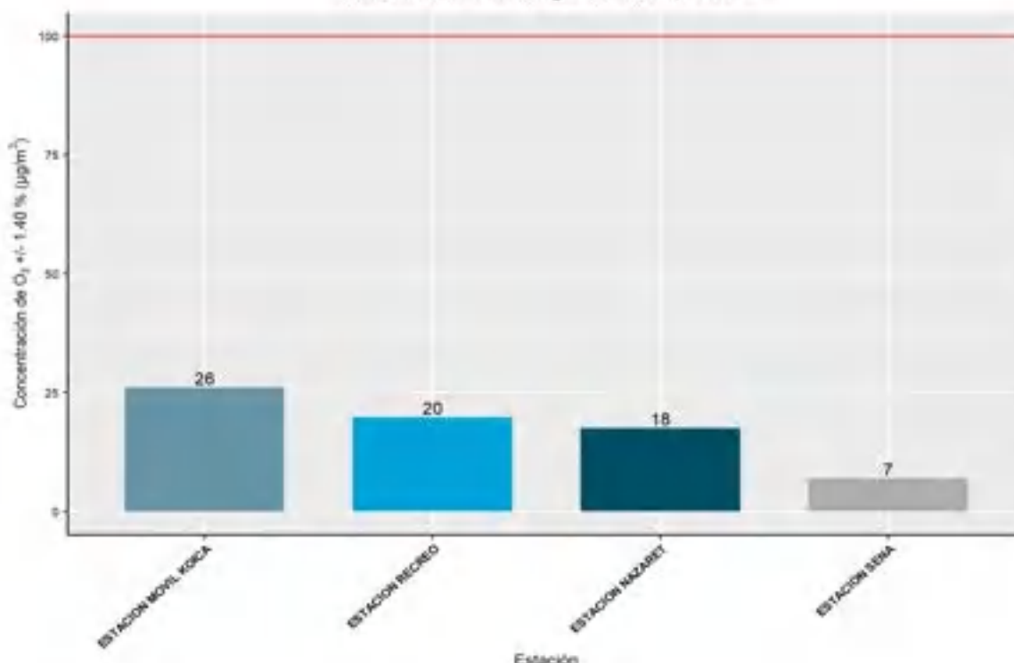
Figura 8. Promedio mensual O 3 Red de monitoreo de calidad del aire CORPOBOYACA Concentración de O 3 . ENERO de 2024
