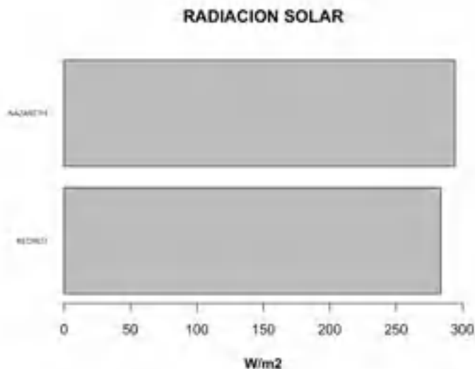
Figura 79. Radiación Solar registrada en estaciones, enero de 2024
