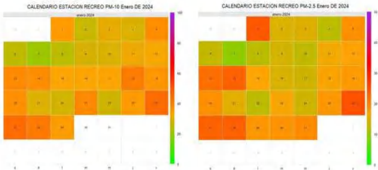
Figura 58. Calendario estación Recreo, enero de 2024
