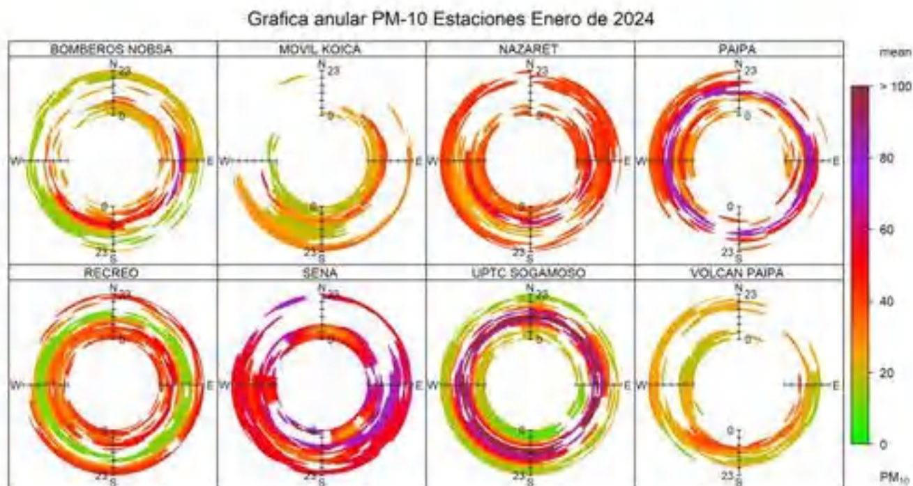
Figura 52. Gráfico anular PM-10 estaciones, enero de 2024
