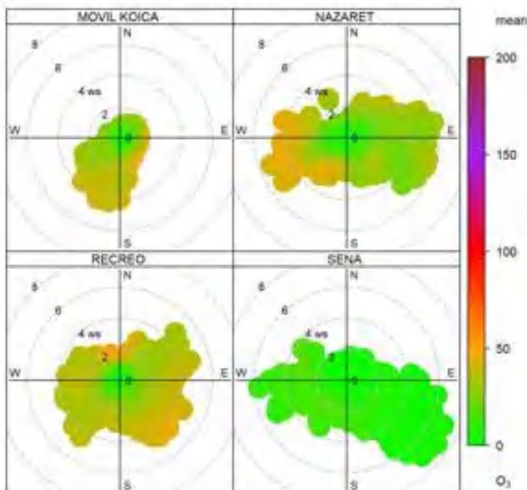
Figura 49. Gráfico Polar por estaciones O 3 , enero de 2024 Grafica Polar O 3 Estaciones Enero de 2024
