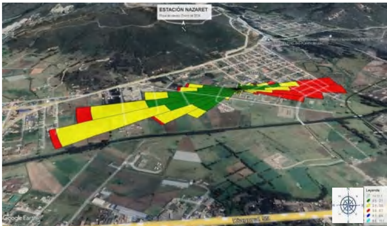
Figura 29. Rosa de vientos estación Nazaret, enero de 2024 (De dónde vienen los vientos)
