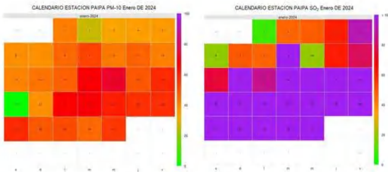
Figura 61. Calendario estación Paipa, enero de 2024
