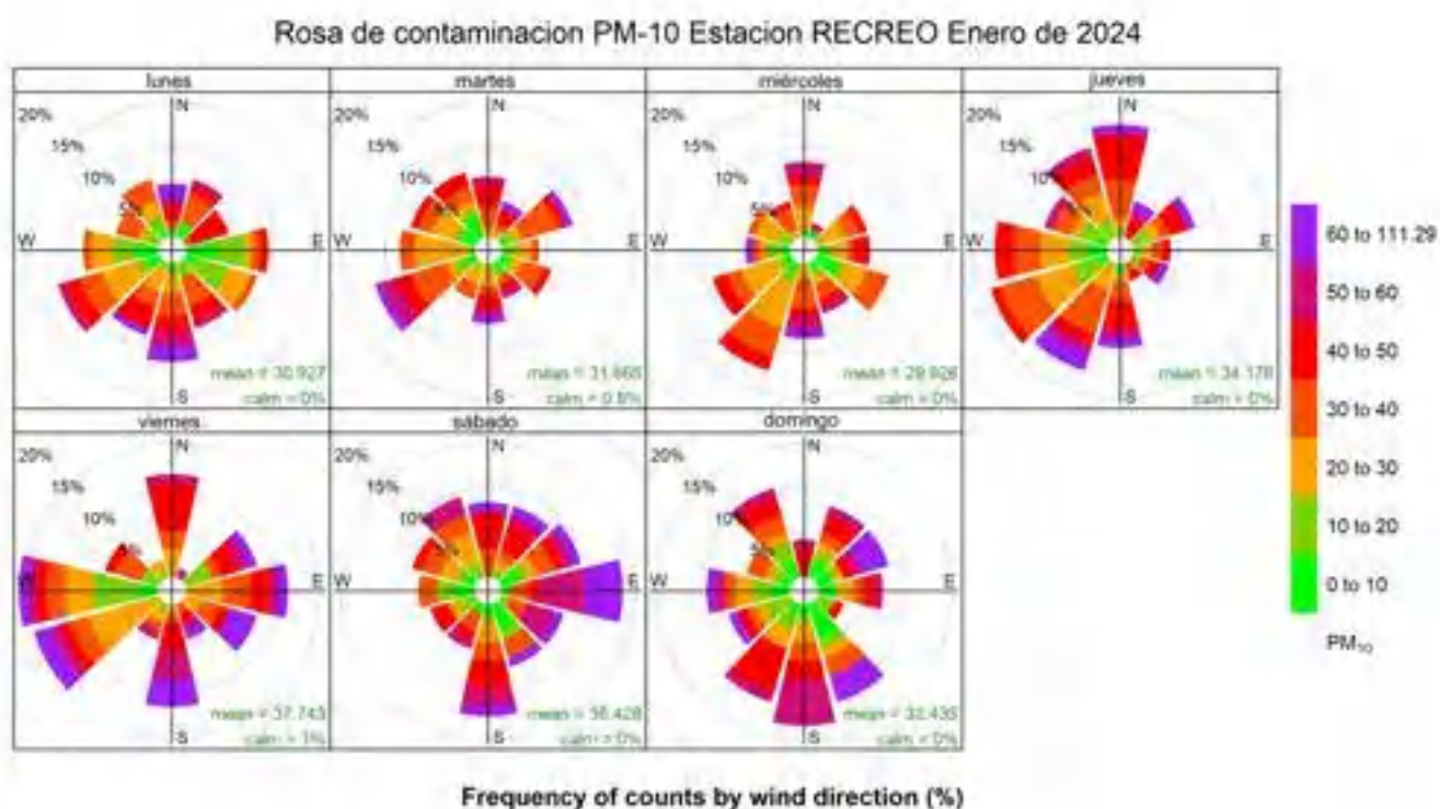
Figura 35. Rosa de contaminación PM-10 estación Recreo, enero de 2024
