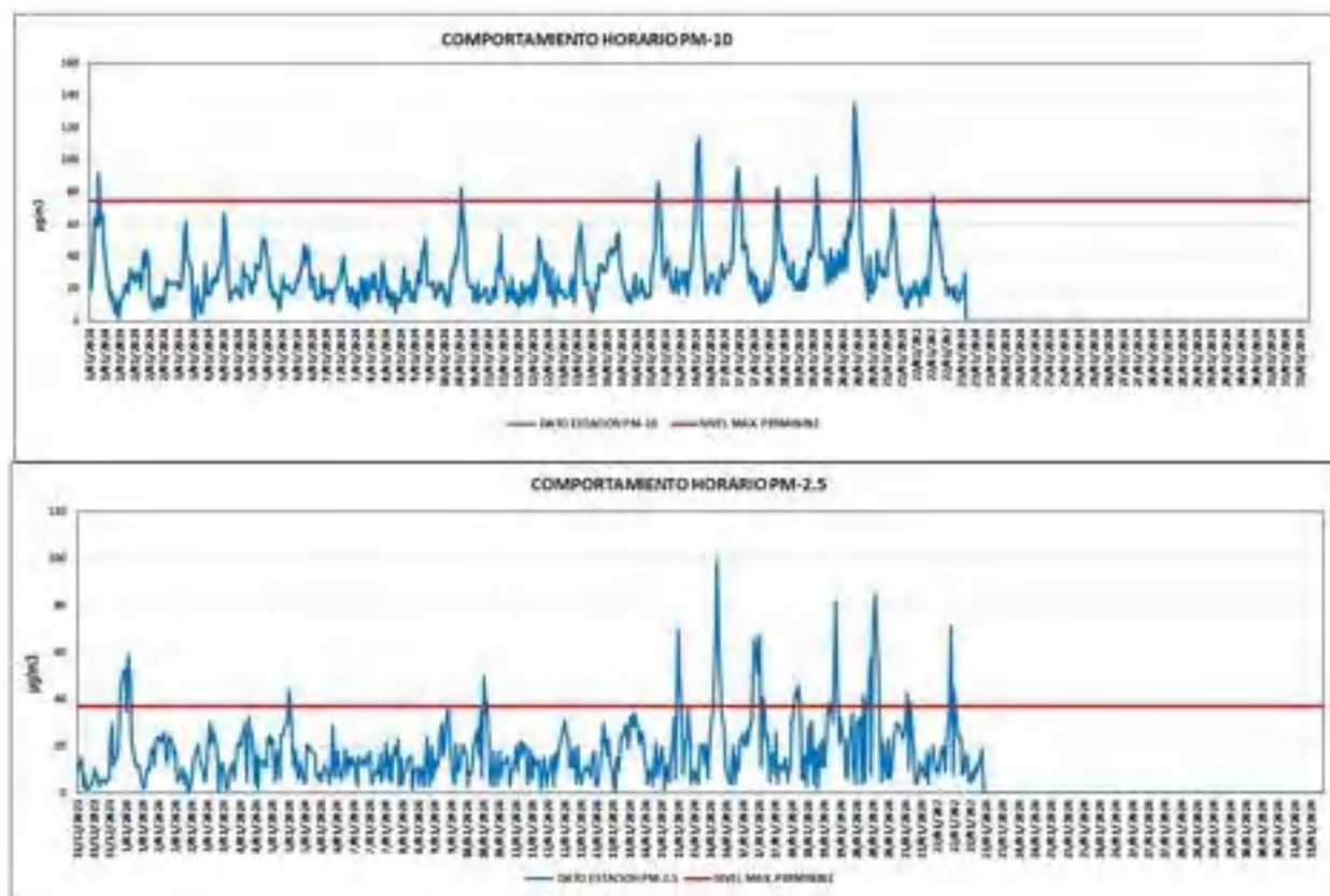
Figura 69. Comportamiento horario PM-10 y PM-2.5 enero de 2024
