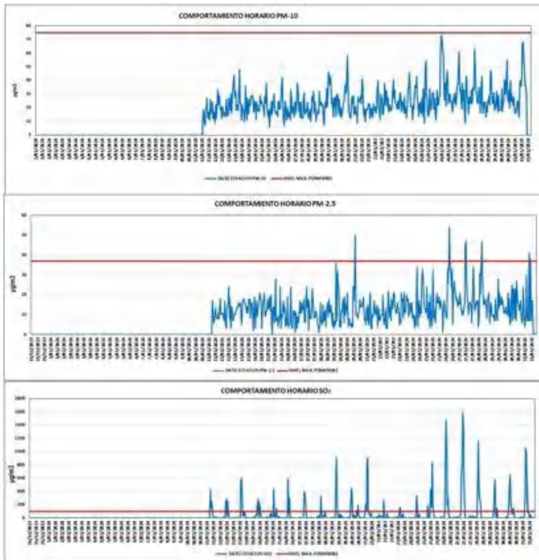
Figura 68. Comportamiento horario PM-10, PM-2.5, y SO 2 enero de 2024
