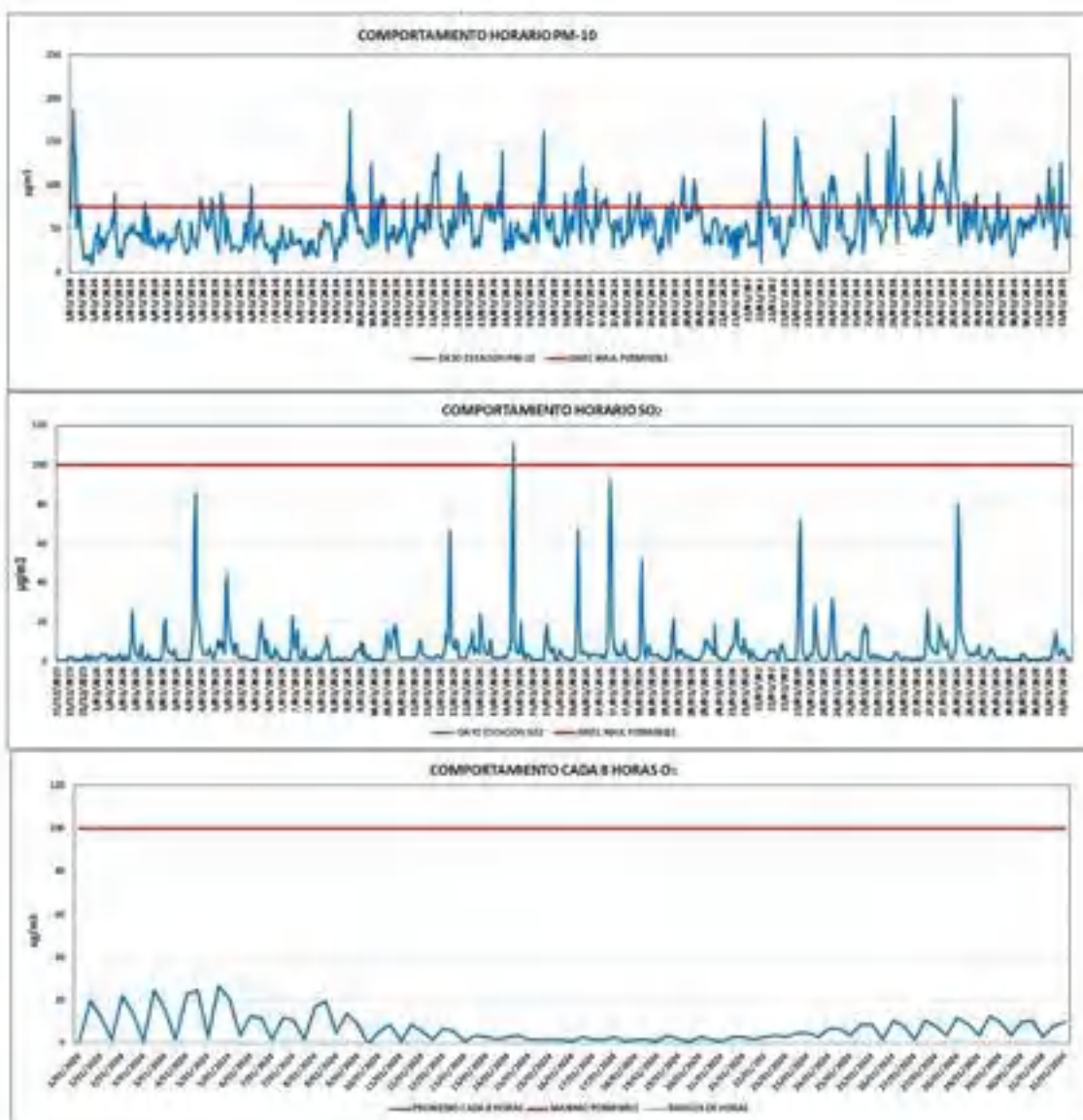
Figura 70. Comportamiento horario PM-10, SO 2 y O 3 , enero de 2024
