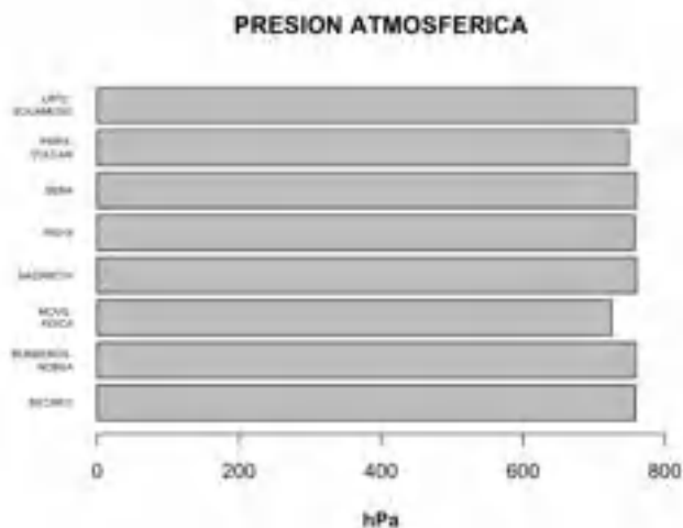
Figura 78. Presión atmosférica registrada en estaciones, enero de 2024
