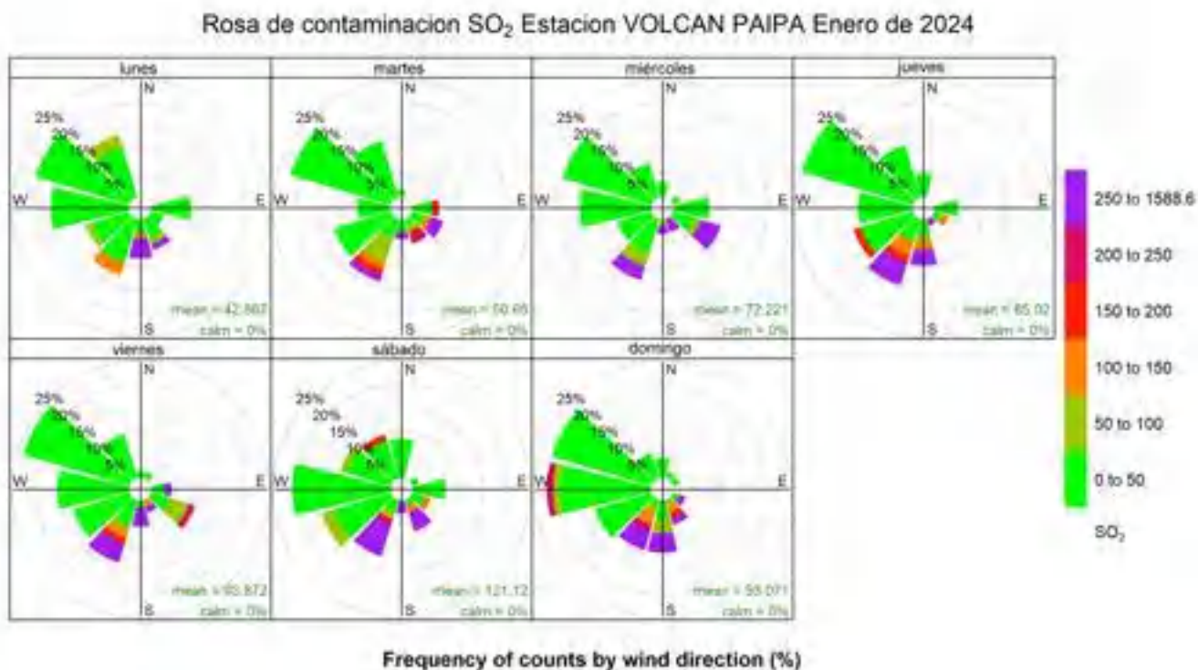
Figura 43. Rosa de contaminación Dióxido de Azufre SO 2 estación volcán Paipa, enero de 2024
