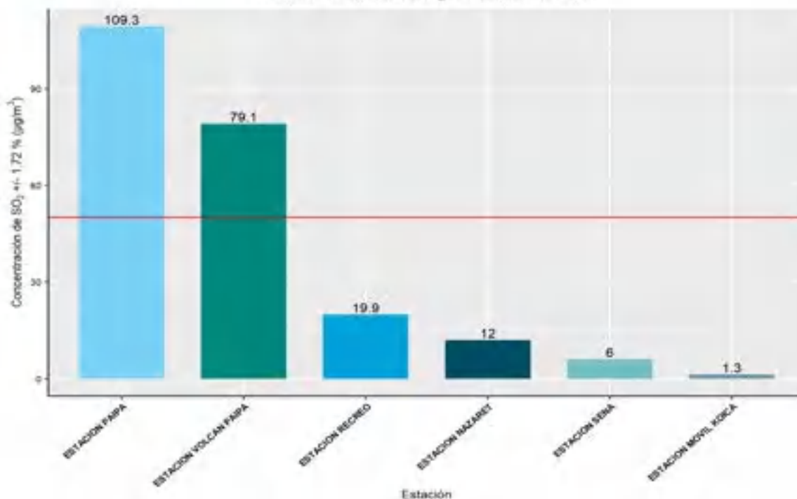
Figura 5. Promedio mensual SO 2 Red de monitoreo de calidad del aire CORPOBOYACA Concentración de SO 2 , ENERO de 2024
