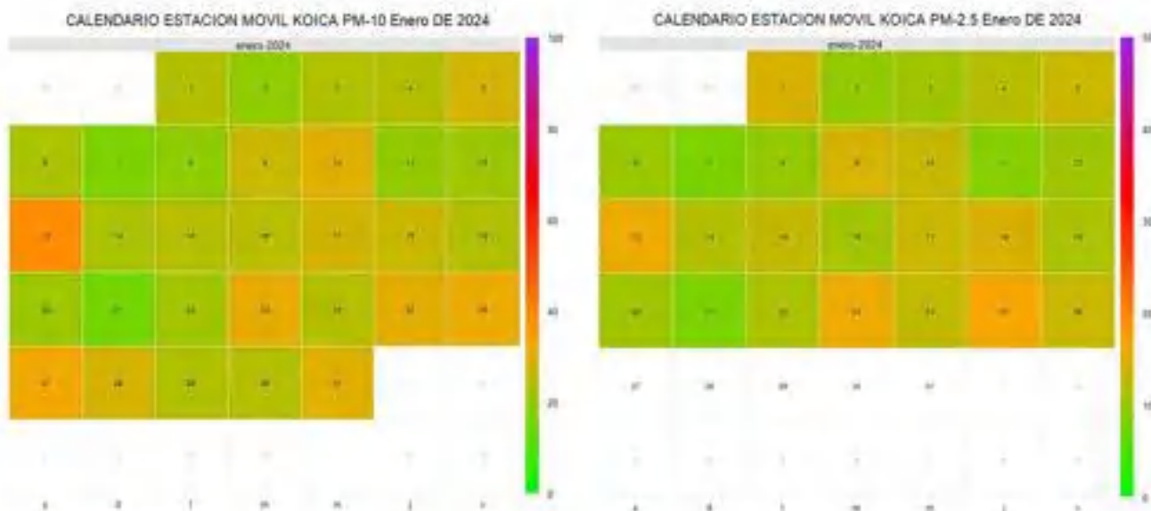
Figura 64. Calendario estación Móvil Koica, enero de 2024
