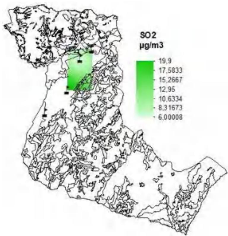
Figura 6. Promedio mensual SO 2 Valle de Sogamoso
