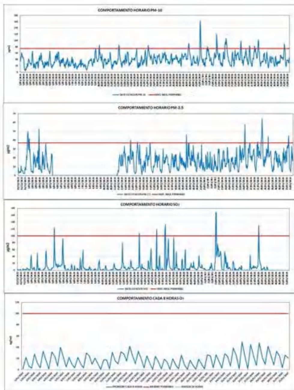
Figura 67. Comportamiento horario PM-10, PM-2.5, SO 2 y O 3 enero de 2024
