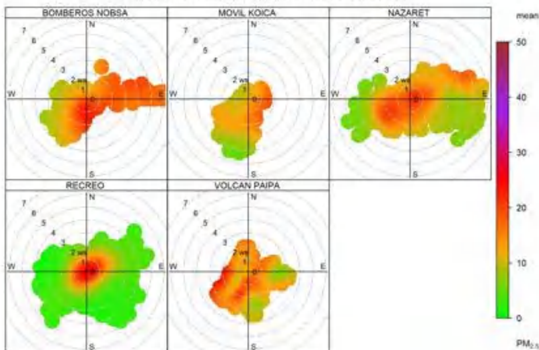
Grafica Polar PM-2.5 Estaciones Enero de 2024
