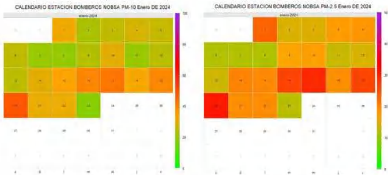
Figura 62. Calendario estación Bomberos Nobsa, enero de 2024
