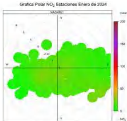
Figura 51. Gráfico Polar por estaciones NO 2 , enero de 2024
