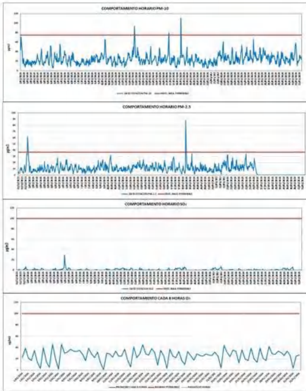
Figura 73. Comportamiento horario PM-10, PM-2.5, SO 2 y O 3 enero de 2024
