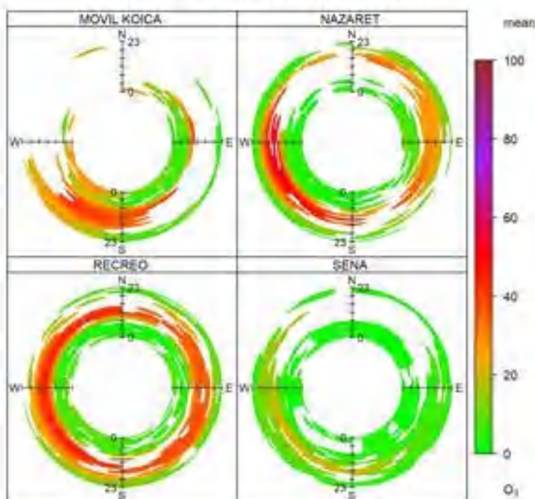
Figura 55. Gráfico anular O 3 estaciones, enero de 2024 Gráfica anular O 3 Estaciones Enero de 2024
