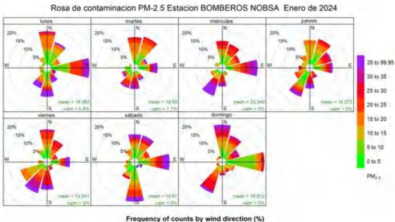
Figura 40. Rosa de contaminación PM-2.5 estación Bomberos Nobsa, enero de 2024
