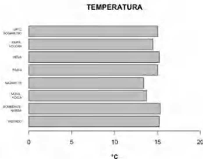
Figura 75. Temperatura registrada en estaciones, enero de 2024
