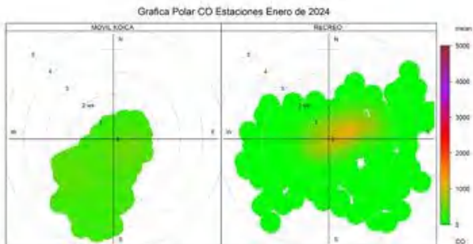
Figura 50. Gráfico Polar por estaciones CO, enero de 2024
