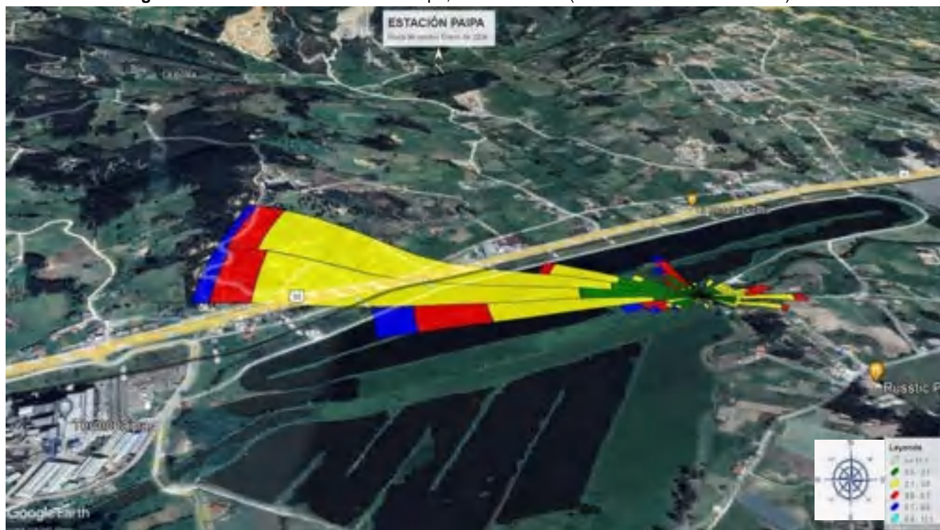
Figura 31. Rosa de vientos estación Paipa, enero de 2024 (De dónde vienen los vientos)
