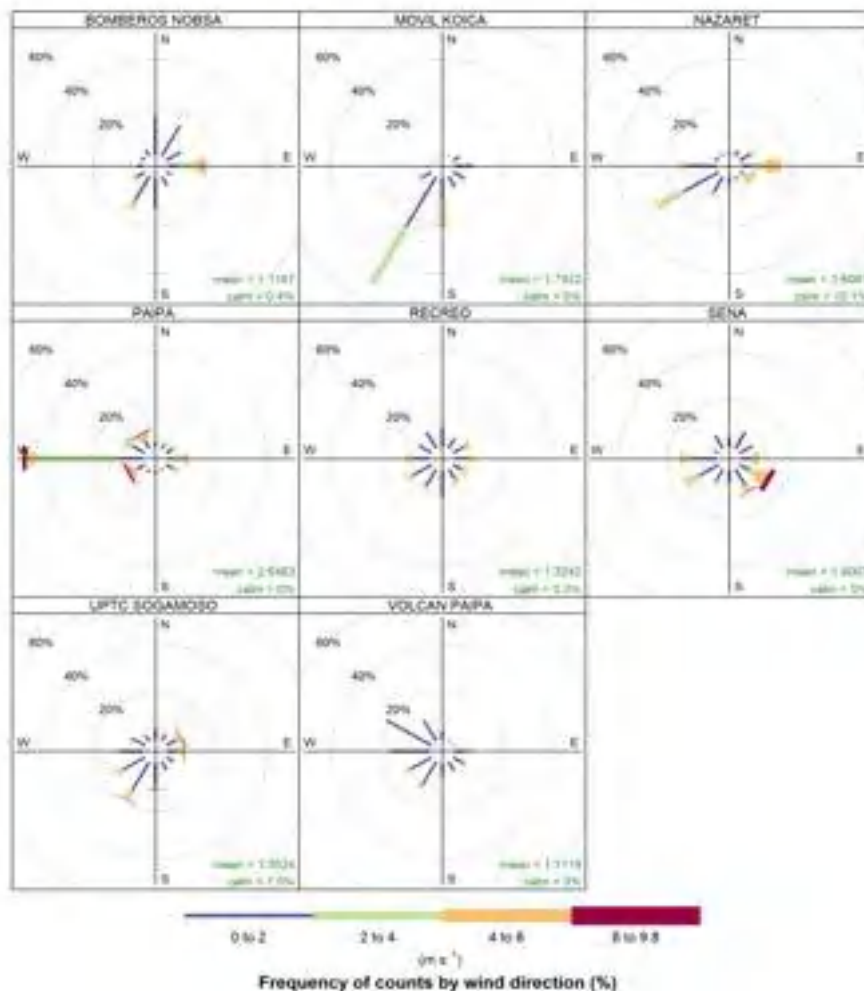
Figura 74. Velocidad y dirección del viento por estaciones enero de 2024
