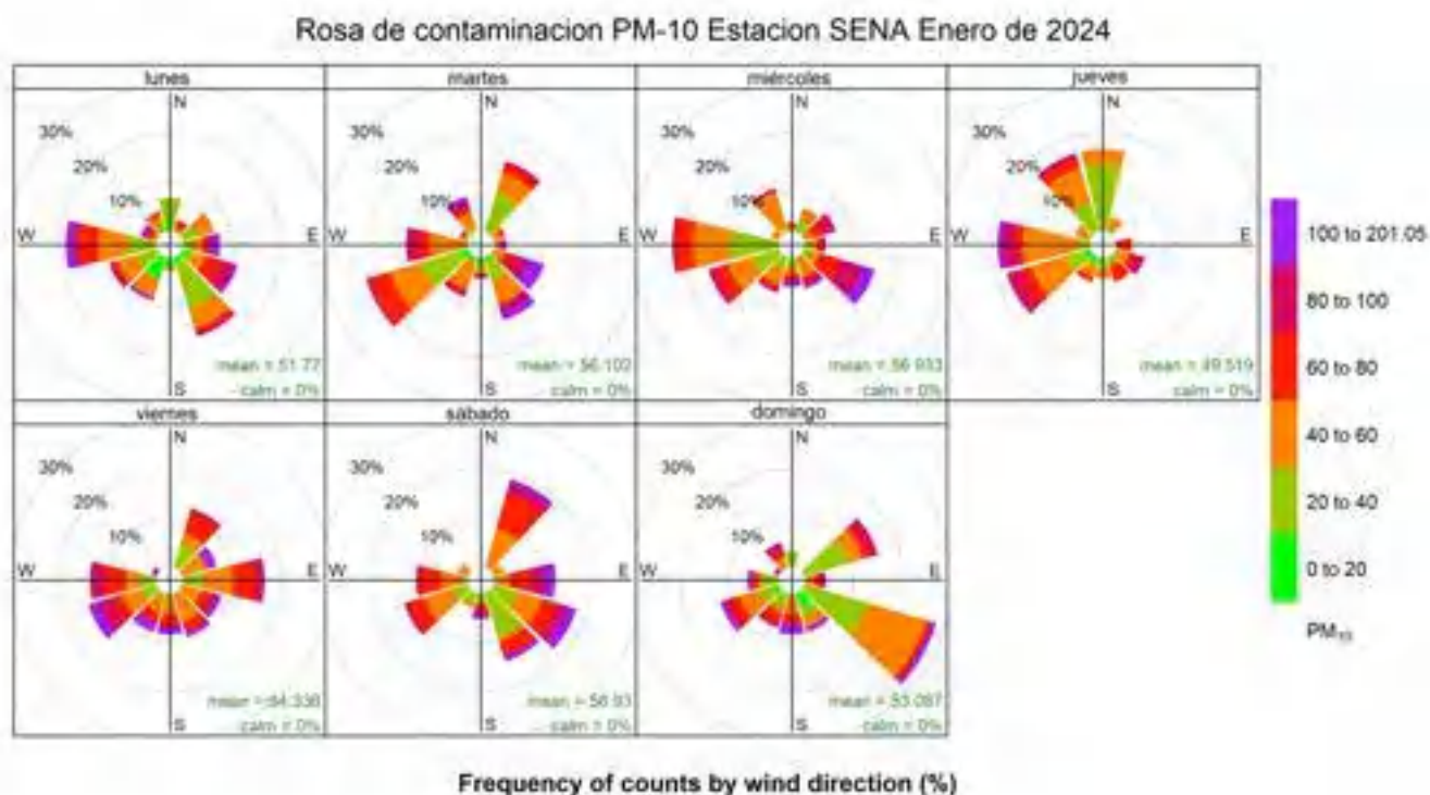
Figura 36. Rosa de contaminación PM-10 estación SENA, enero de 2024
