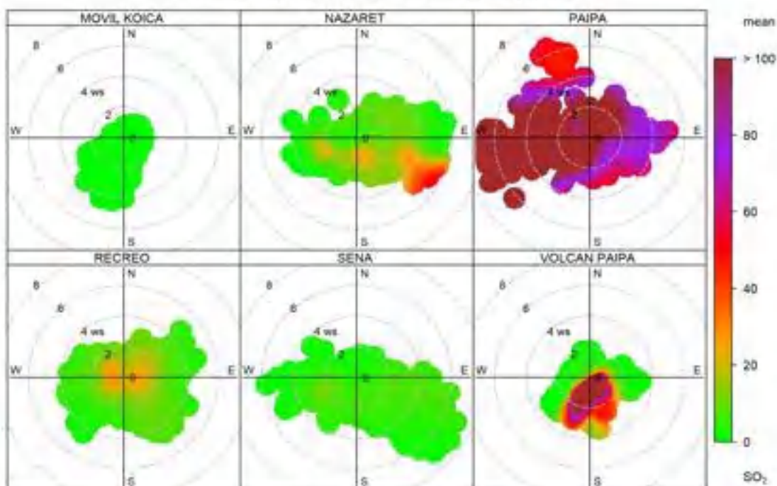
Figura 48. Gráfico Polar por estaciones SO 2 , enero de 2024 Gráfica Polar SO 2 Estaciones Enero de 2024
