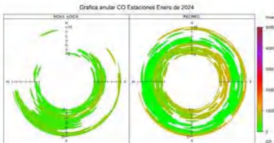
Figura 56. Gráfico anular CO estaciones, enero de 2024
