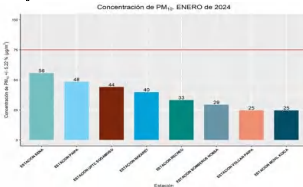
Figura 1. Promedio mensual PM-10 Red de monitoreo de calidad del aire CORPOBOYACA
