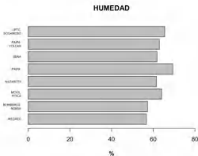
Figura 77. Humedad registrada en las estaciones, enero de 2024
