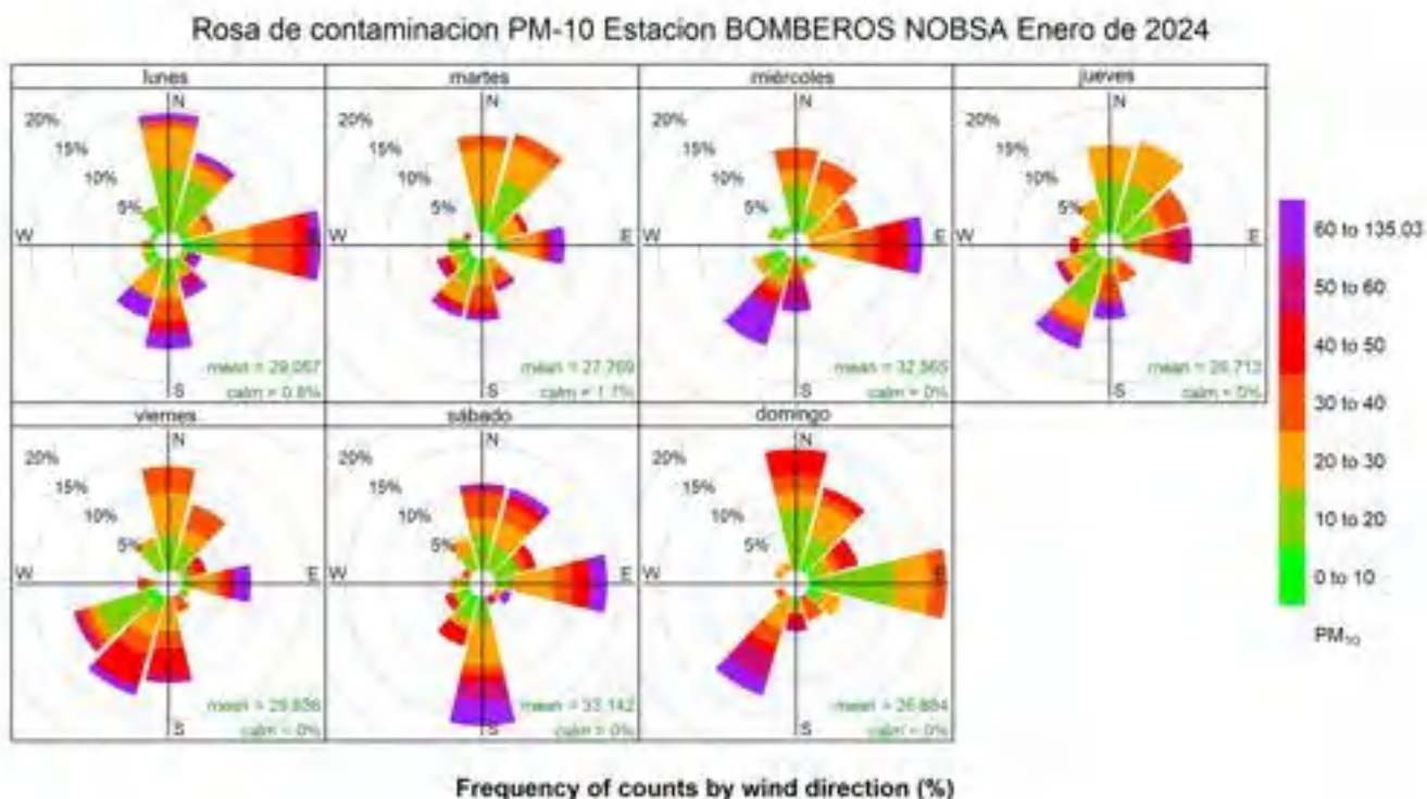
Figura 39. Rosa de contaminación PM-10 estación Bomberos Nobsa, enero de 2024
