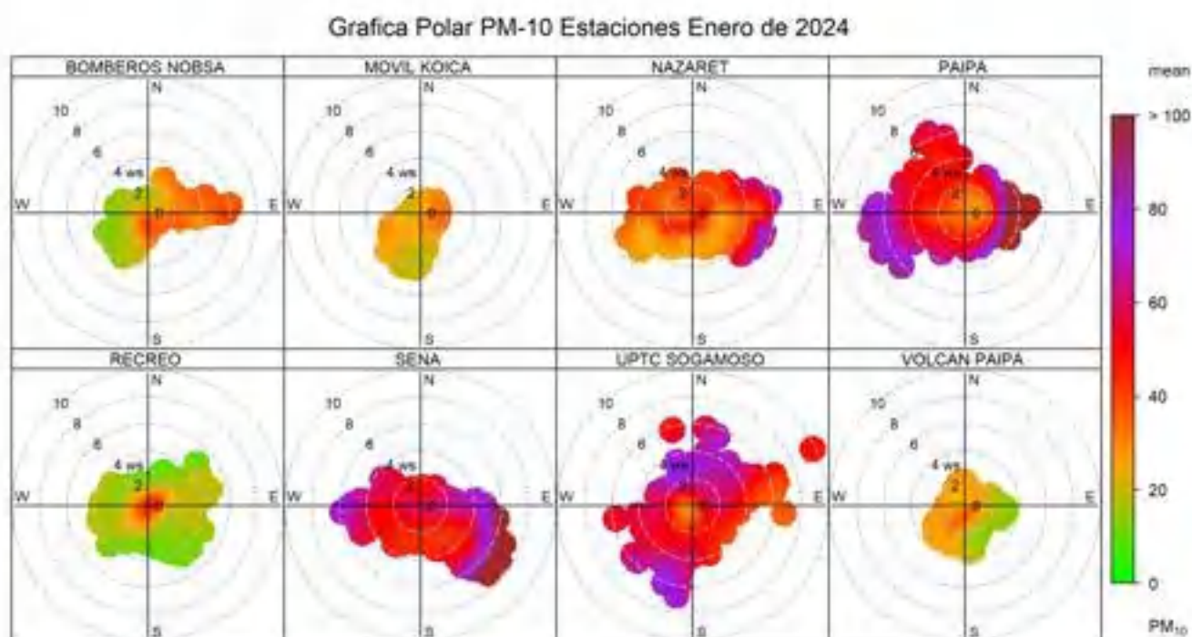
Figura 46. Gráfico polar por estaciones PM-10, enero de 2024
