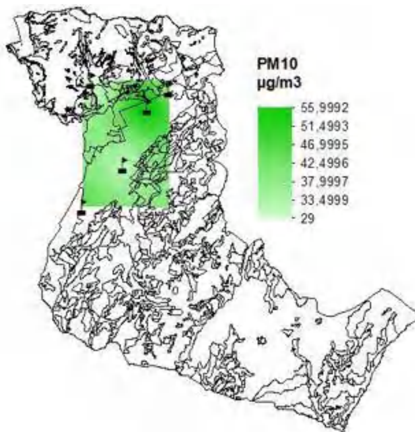
Figura 2. Promedio mensual PM-10 Valle de Sogamoso
