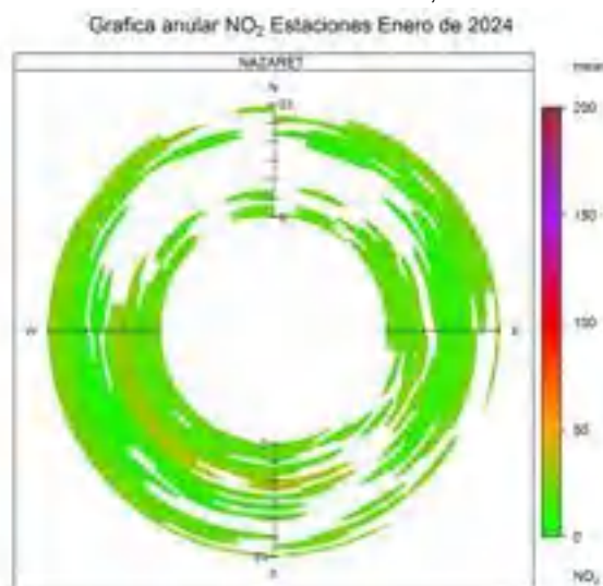
Figura 57. Gráfico anular NO 2 estaciones, enero de 2024
