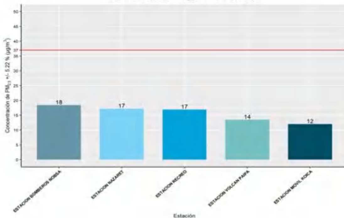
Figura 3. Promedio mensual PM-2.5 Red de monitoreo de calidad del aire CORPOBOYACA Concentración de PM 2.5 . ENERO de 2024
