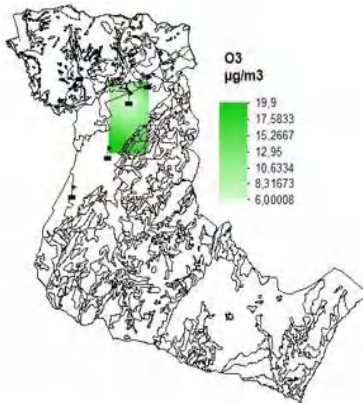
Figura 9. Promedio mensual O 3 Valle de Sogamoso
