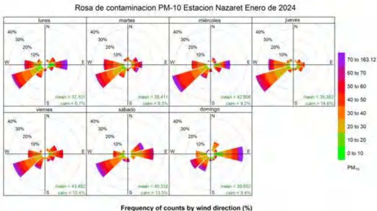
Figura 41. Rosa de contaminación PM-10 estación Nazaret, enero de 2024
