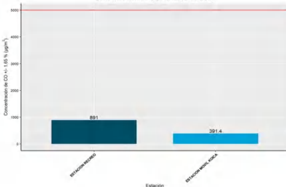
Figura 10. Promedio mensual CO Red de monitoreo de calidad del aire CORPOBOYACA Concentración de CO. ENERO de 2024
