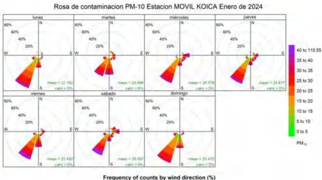
Figura 45. Rosa de contaminación PM-10 estación Móvil Koica, enero de 2024
