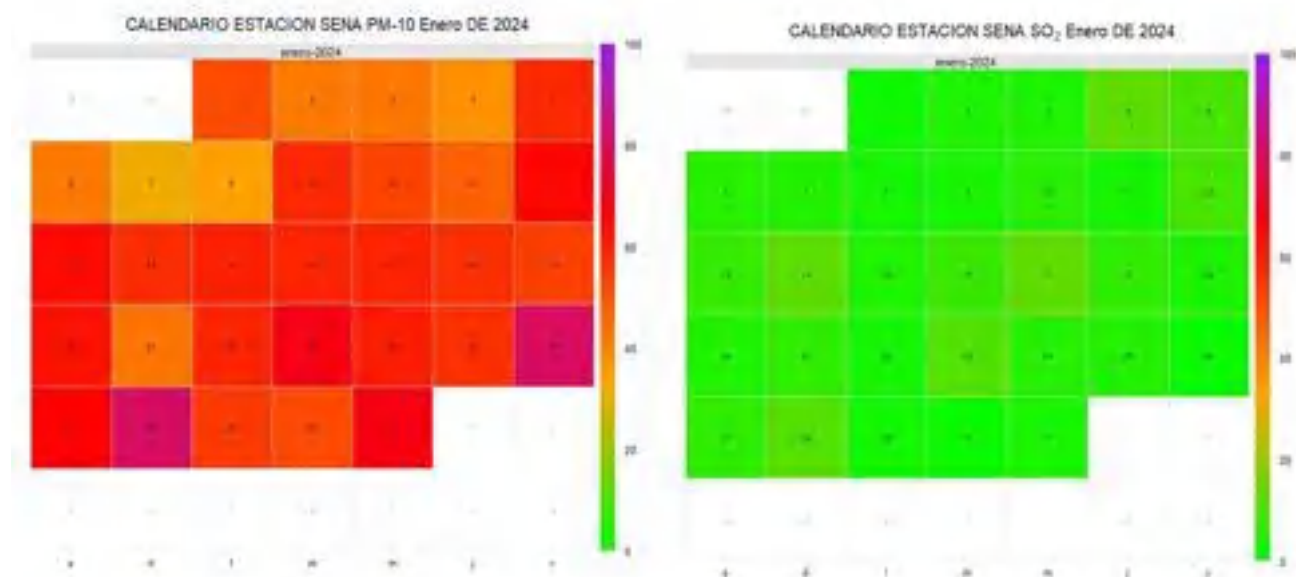
Figura 59. Calendario estación SENA, enero de 2024
