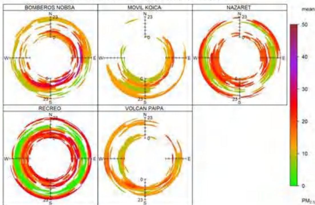
Grafica anular PM-2.5 Estaciones Enero de 2024
