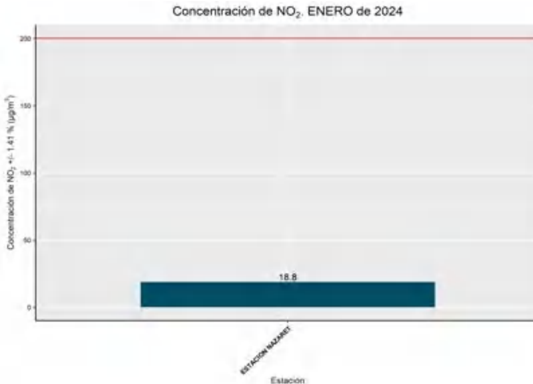
Figura 7. Promedio mensual NO 2 Red de monitoreo de calidad del aire CORPOBOYACA
