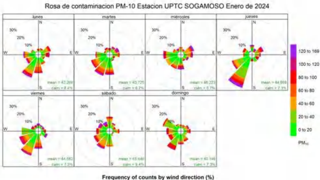
Figura 44. Rosa de contaminación PM-10 estación UPTC Sogamoso, enero de 2024
