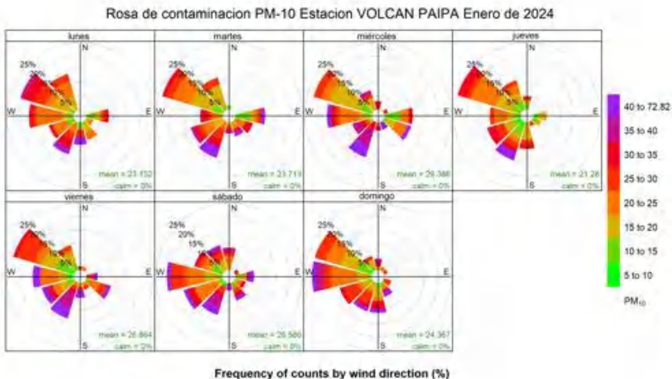
Figura 42. Rosa de contaminación PM-10 estación volcán Paipa, enero de 2024
