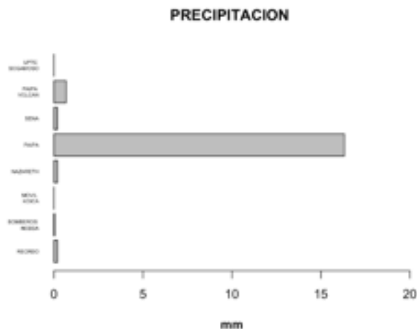
Figura 76. Precipitación registrada en las estaciones, enero de 2024
