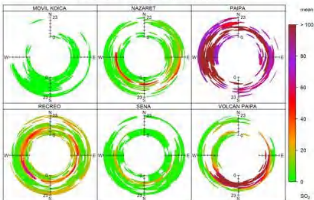
Figura 54. Gráfico anular SO 2 estaciones, enero de 2024 Grafica anular SO 2 Estaciones Enero de 2024
