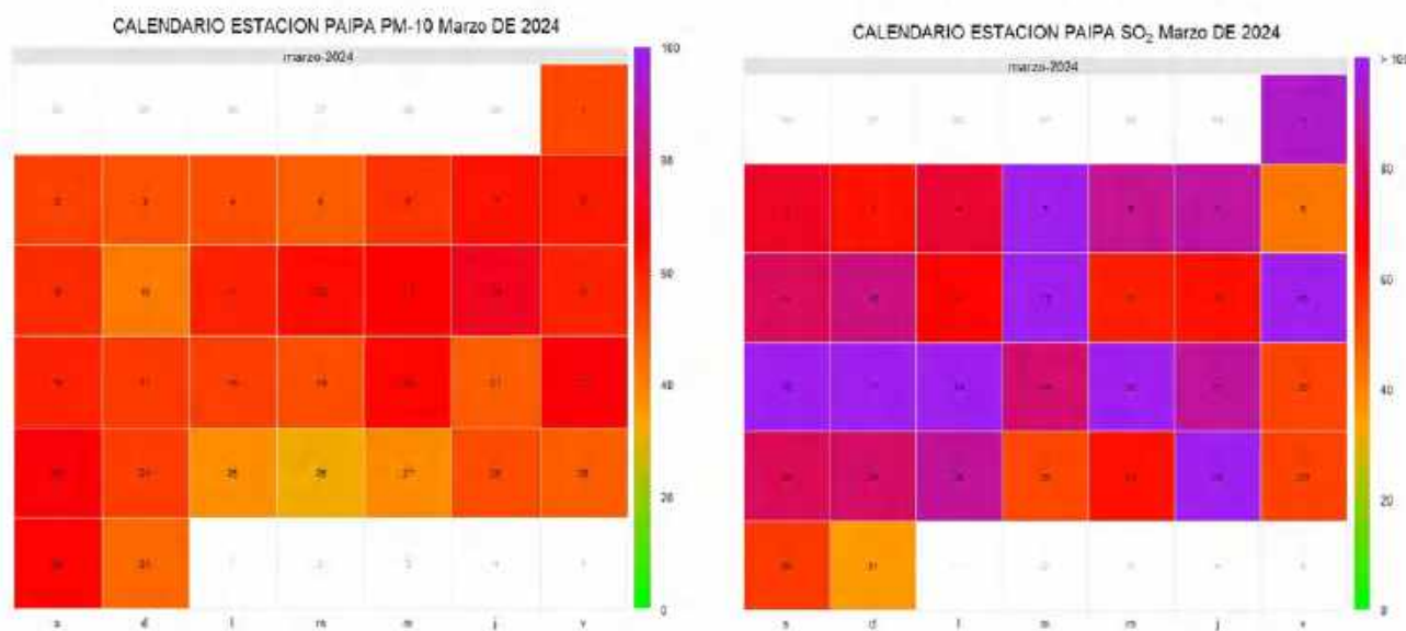
Figura 61. Calendario estación Paipa, marzo de 2024
