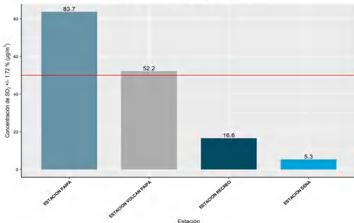
Figura 5. Promedio mensual SO 2 Red de monitoreo de calidad del aire CORPOBOYACA Concentración de SO 2 . MARZO de 2024
