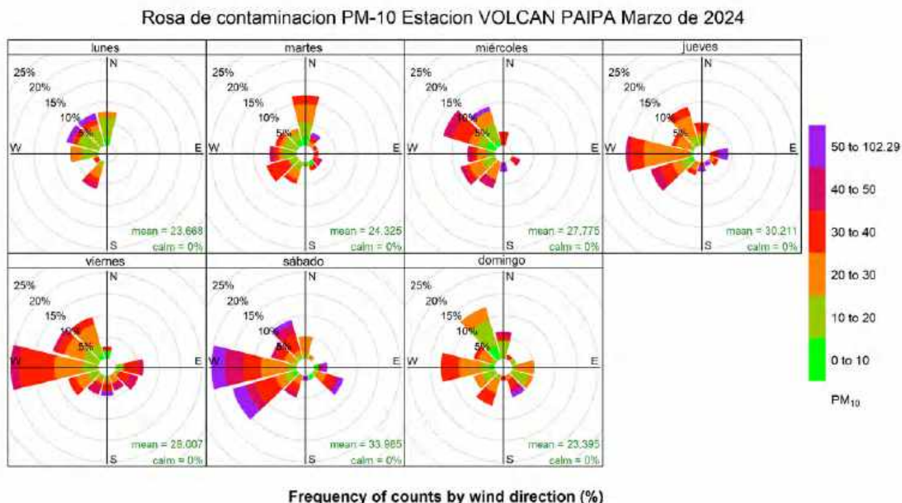
Figura 42. Rosa de contaminación PM-10 estación volcán Paipa, marzo de 2024
