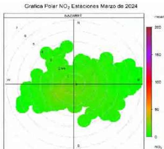
Figura 51. Gráfico Polar por estaciones NO 2 , marzo de 2024
