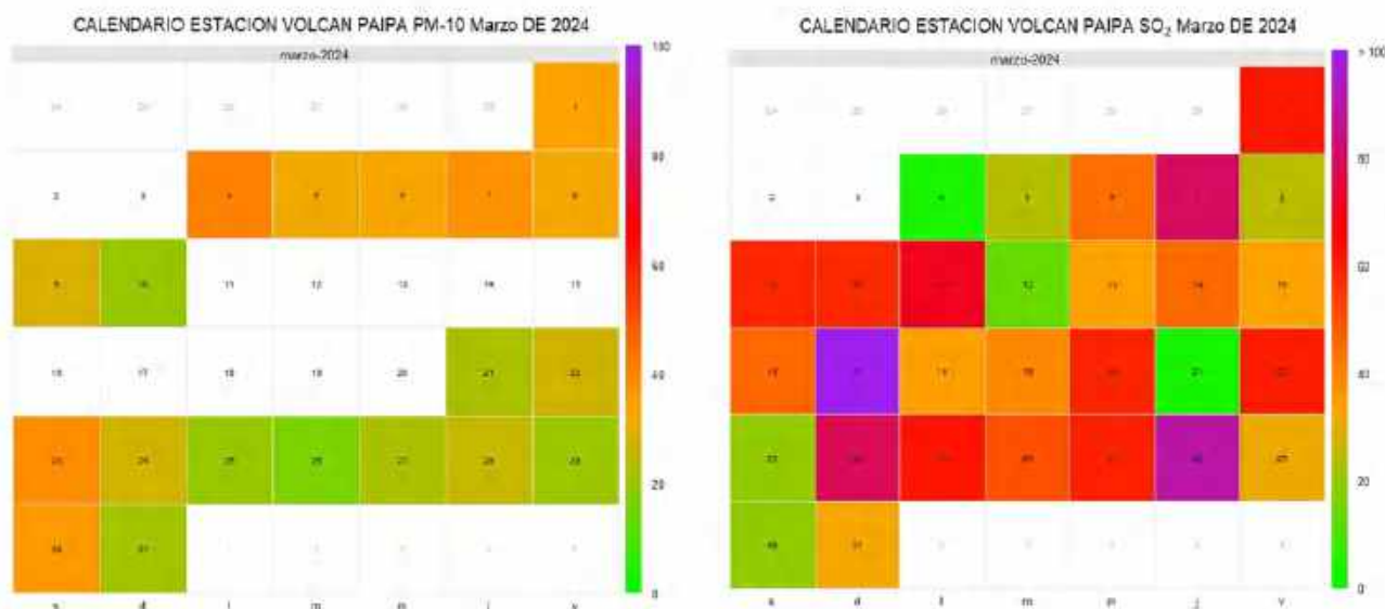
Figura 63. Calendario estación Volcán Paipa, marzo de 2024
