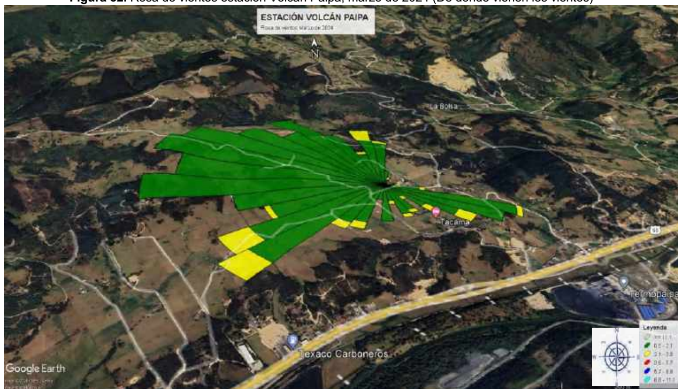
Figura 32. Rosa de vientos estación Volcán Paipa, marzo de 2024 (De dónde vienen los vientos)
