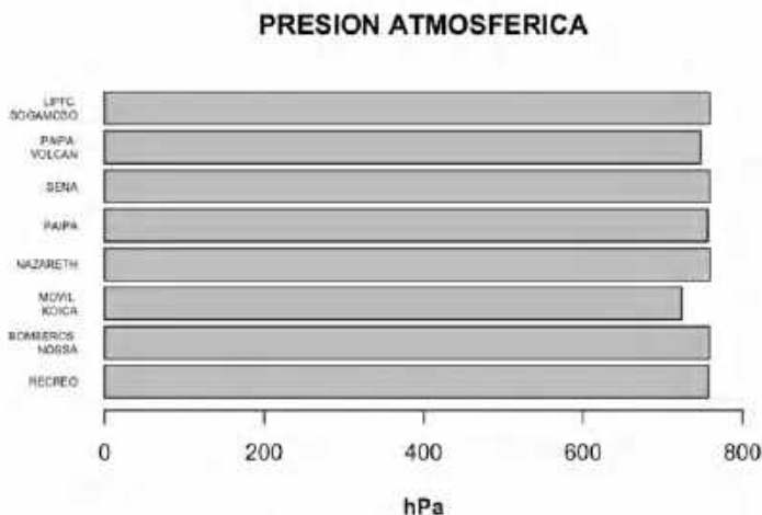
Figura 78. Presión atmosférica registrada en estaciones, marzo de 2024
