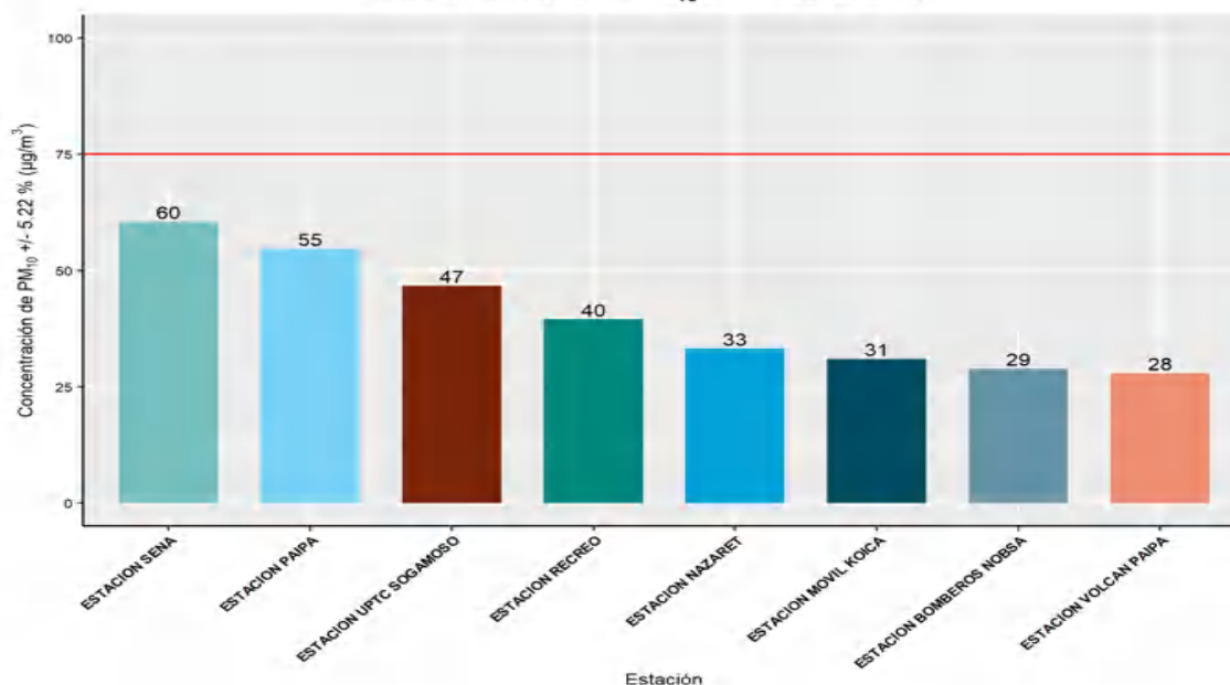
Figura 1. Promedio mensual PM-10 Red de monitoreo de calidad del aire CORPOBOYACA Concentración de PM 10 . MARZO de 2024
