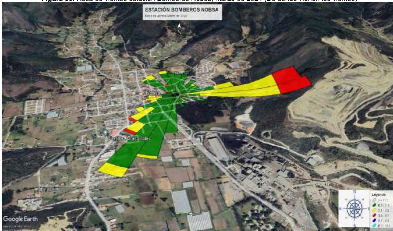
Figura 30. Rosa de vientos estación Bomberos Nobsa, marzo de 2024 (De dónde vienen los vientos)
