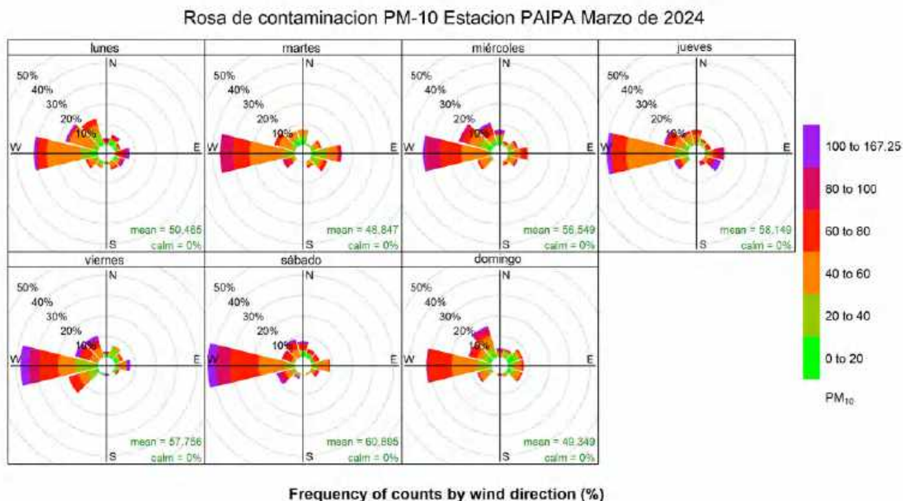
Figura 37. Rosa de contaminación PM-10 estación Paipa, marzo de 2024
