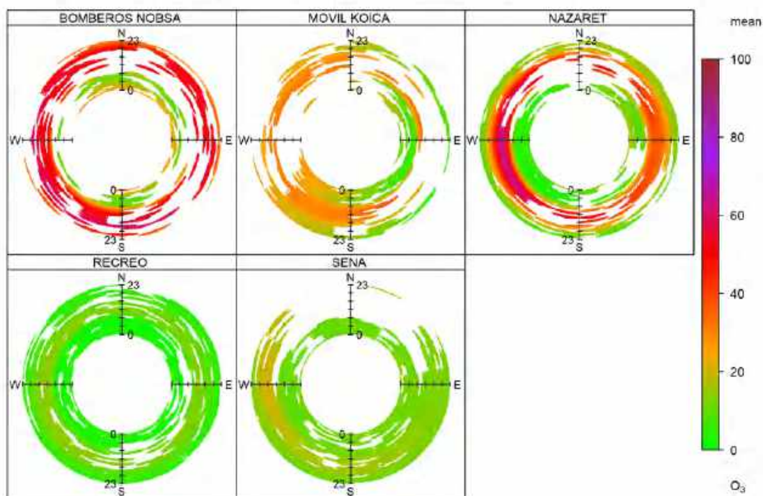
Figura 55. Gráfico anular O 3 estaciones, marzo de 2024 Grafica anular O 3 Estaciones Marzo de 2024
