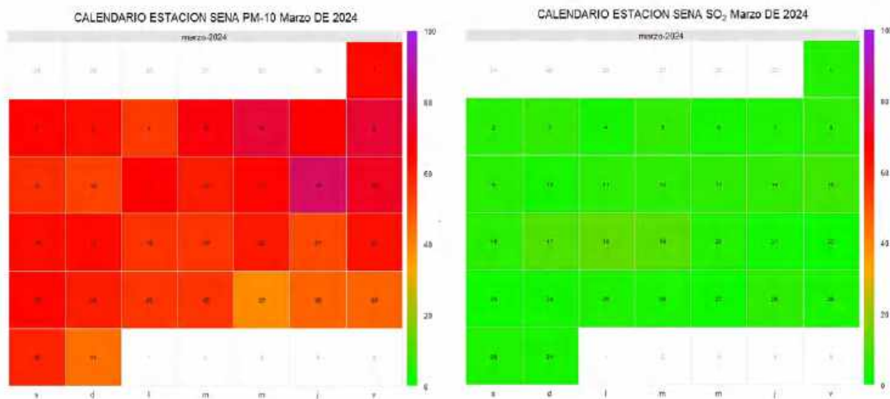
Figura 59. Calendario estación SENA, marzo de 2024
