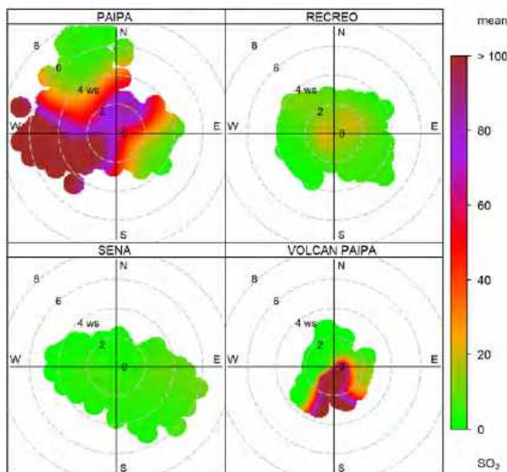
Figura 48. Gráfico Polar por estaciones SO 2 , marzo de 2024 Grafica Polar SO 2 Estaciones Marzo de 2024
