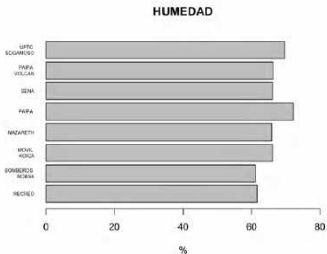
Figura 77. Humedad registrada en las estaciones, marzo de 2024
