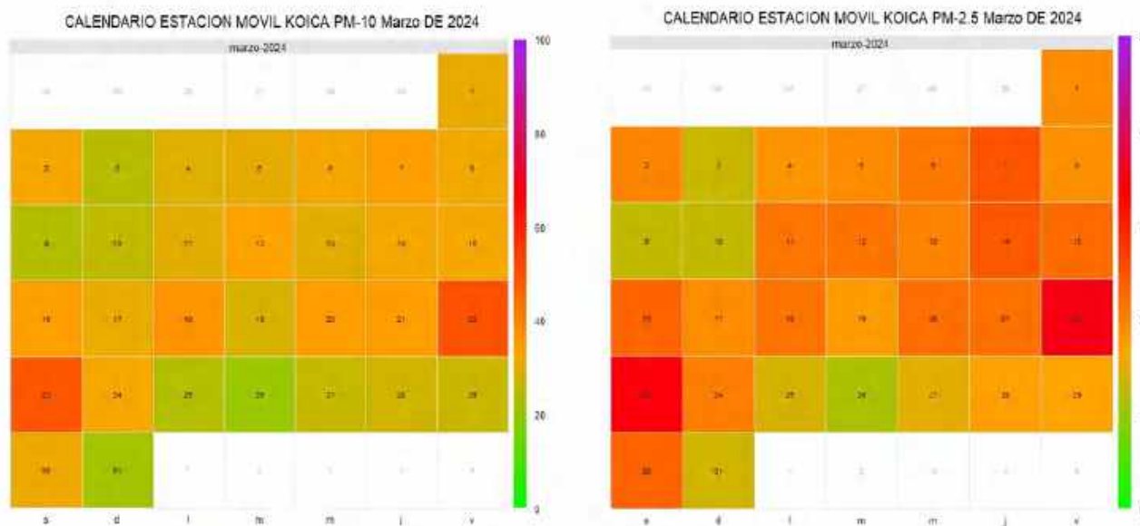
Figura 64. Calendario estación Móvil Koica, marzo de 2024
