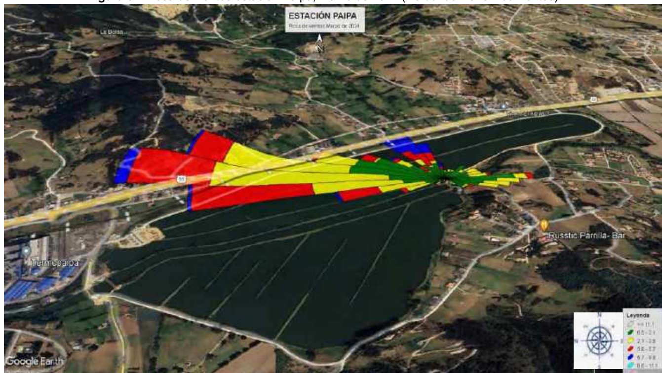
Figura 31. Rosa de vientos estación Paipa, marzo de 2024 (De dónde vienen los vientos)
