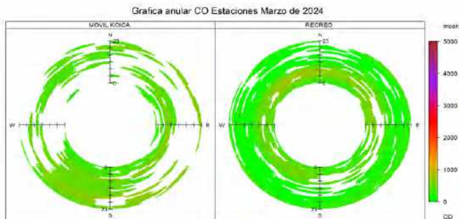
Figura 56. Gráfico anular CO estaciones, marzo de 2024
