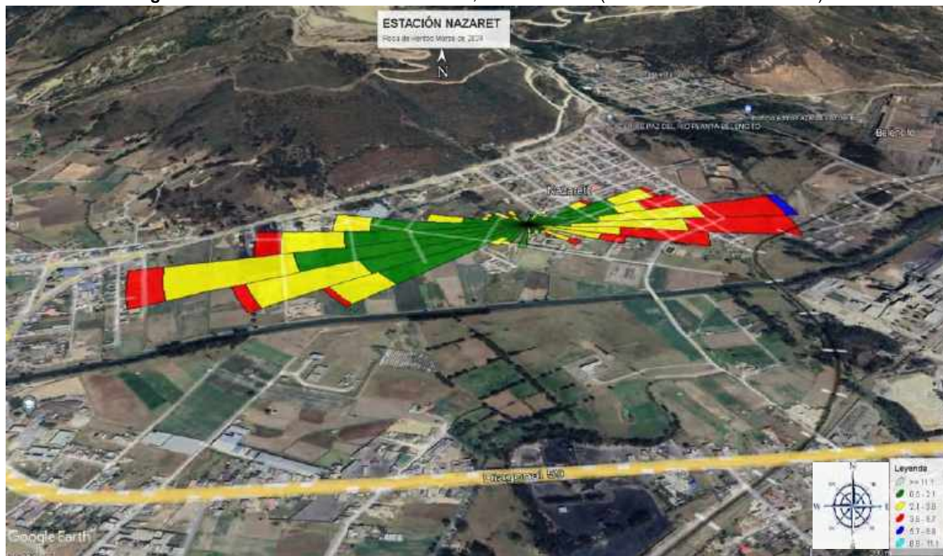
Figura 29. Rosa de vientos estación Nazaret, marzo de 2024 (De dónde vienen los vientos)
