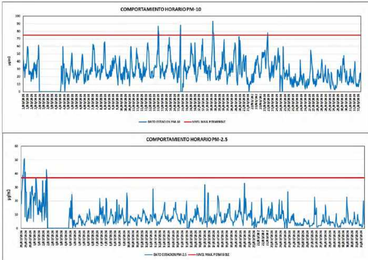
Figura 69. Comportamiento horario PM-10 y PM-2.5 marzo de 2024
