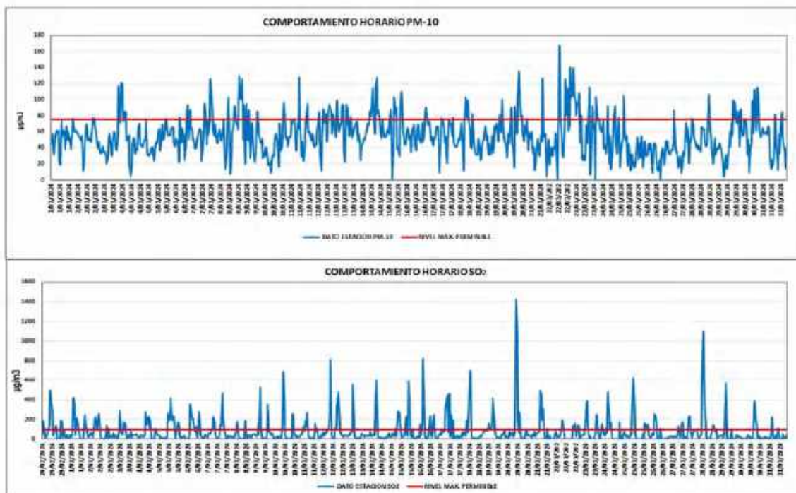
Figura 71. Comportamiento horario PM-10 y SO2, marzo de 2024
