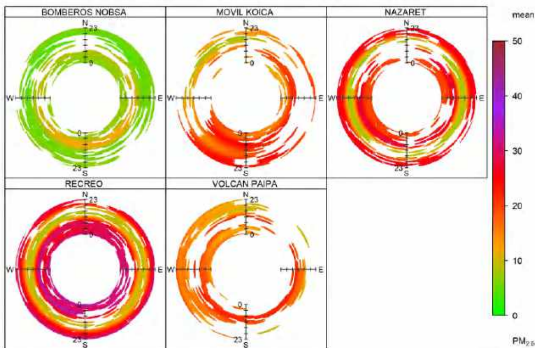
Figura 53. Gráfico anular PM-2.5 estaciones, marzo de 2024 Grafica anular PM-2.5 Estaciones Marzo de 2024
