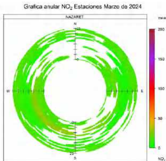
Figura 57. Gráfico anular NO 2 estaciones, marzo de 2024
