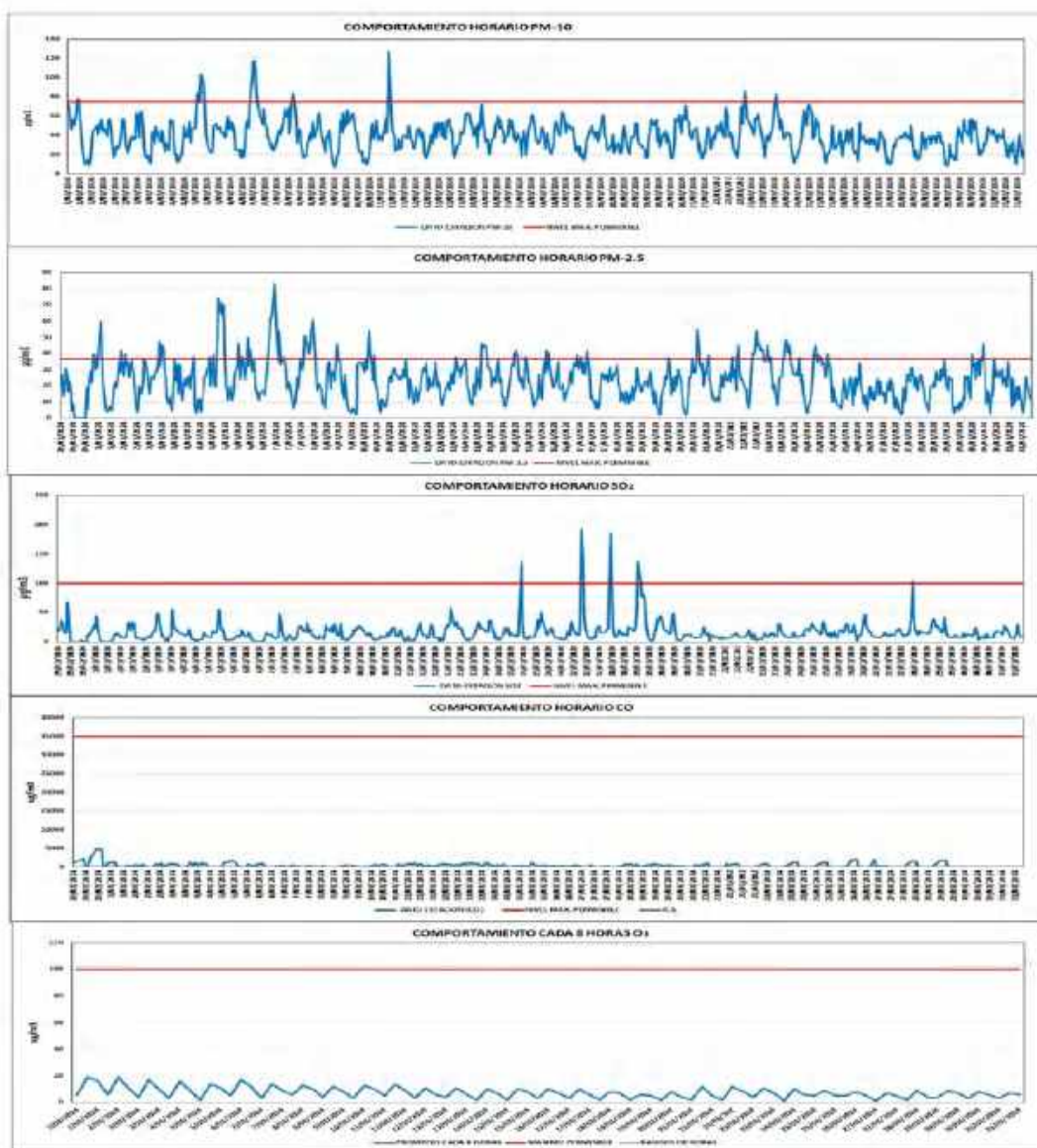
Figura 66. Comportamiento horario PM-10, PM-2.5, SO 2 , CO y O 3 marzo de 2024
