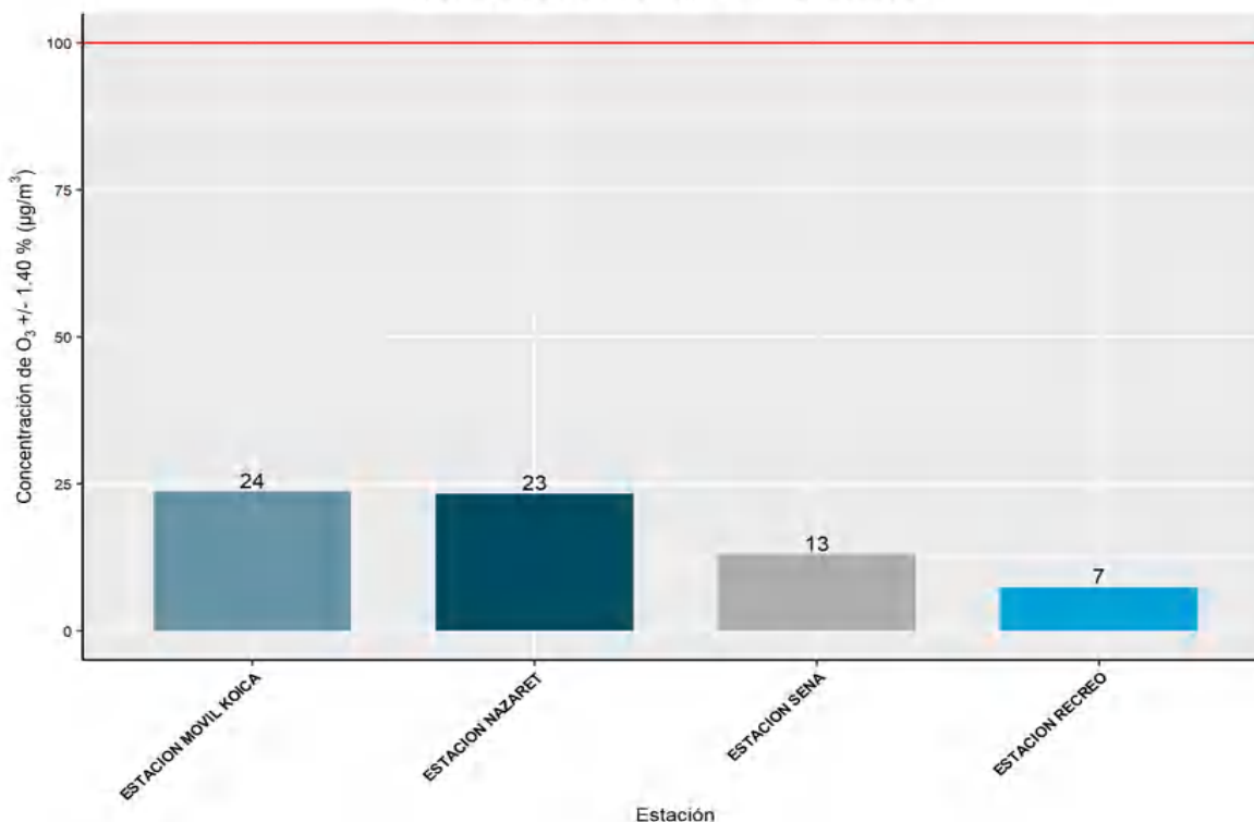
Figura 8. Promedio mensual O 3 Red de monitoreo de calidad del aire CORPOBOYACA Concentración de O 3 . MARZO de 2024
