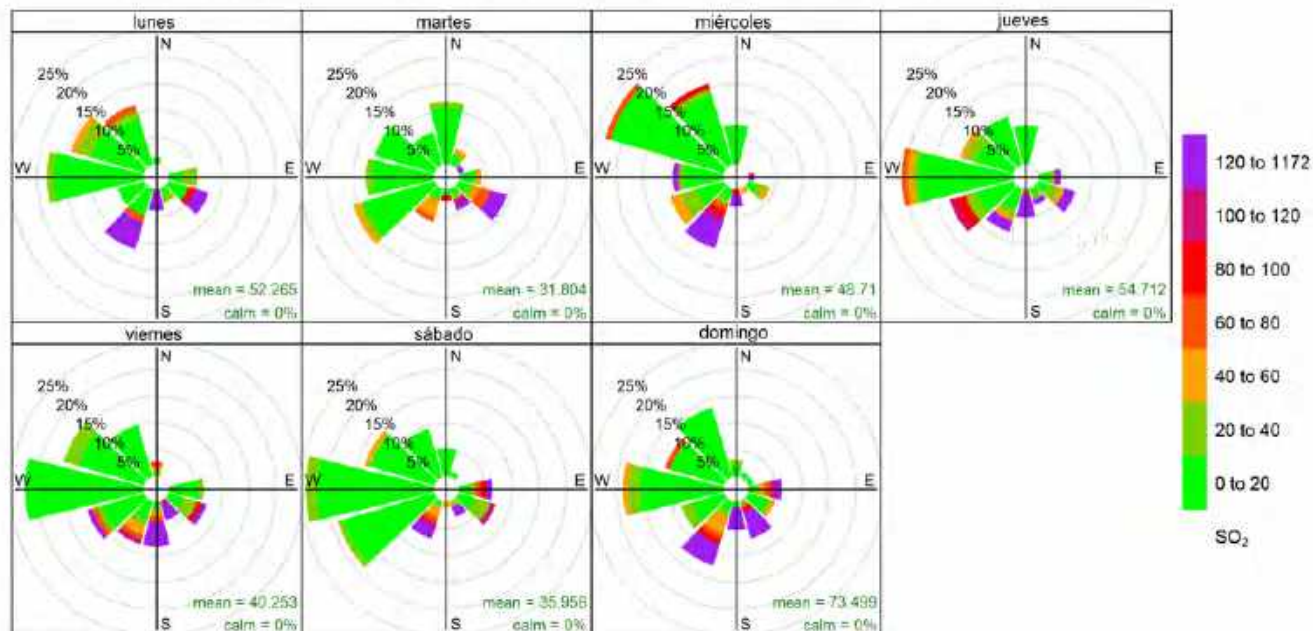
Rosa de contaminación SO 2 Estacion VOLCAN PAIPA Marzo de 2024
