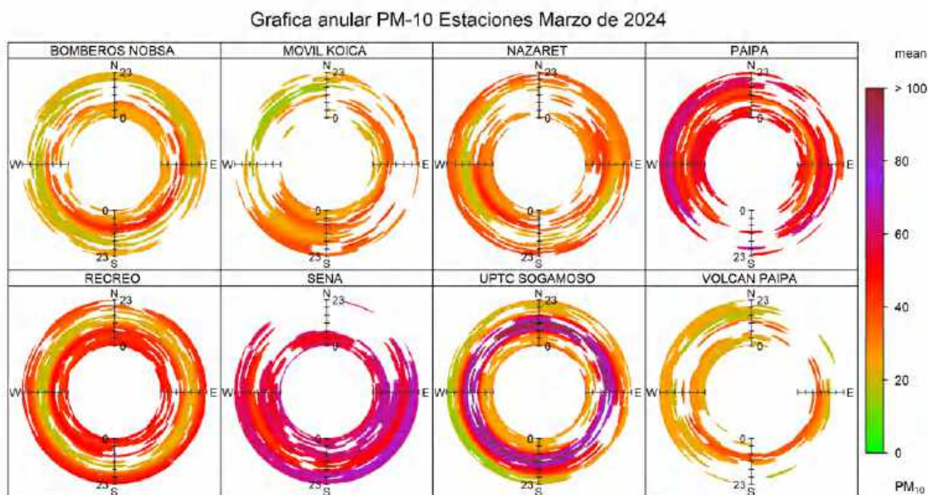
Figura 52. Gráfico anular PM-10 estaciones, marzo de 2024
