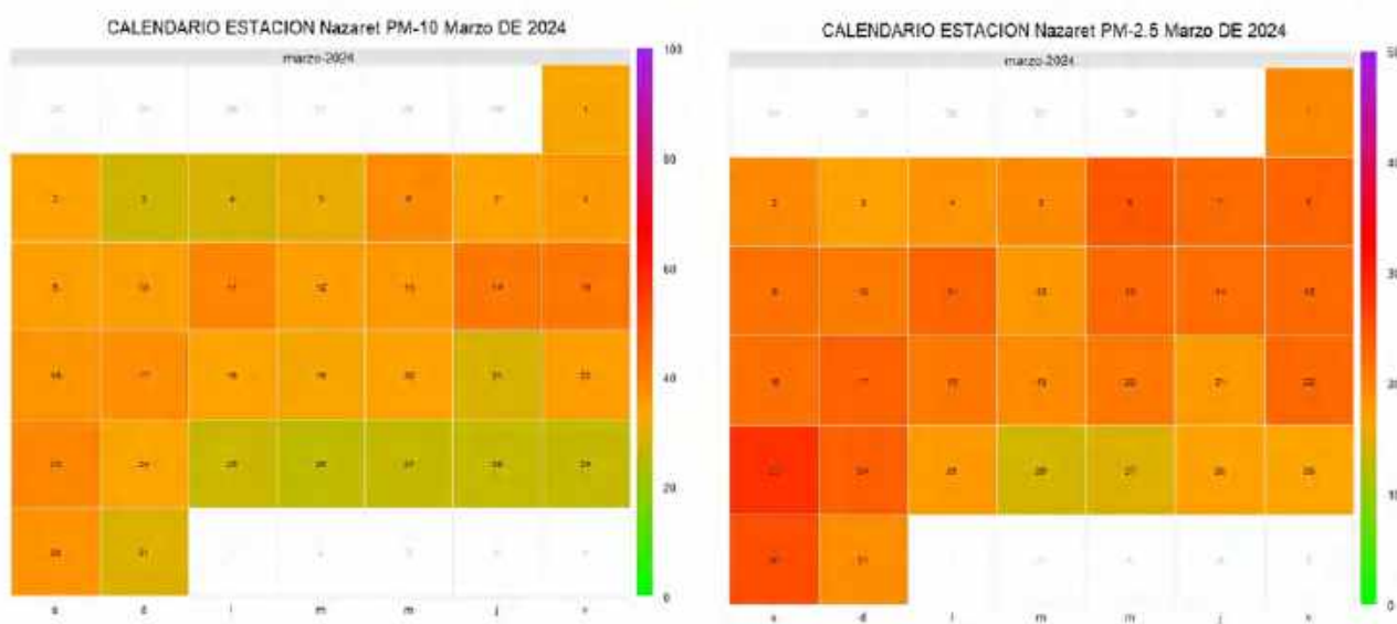
Figura 60. Calendario estación Nazaret, marzo de 2024
