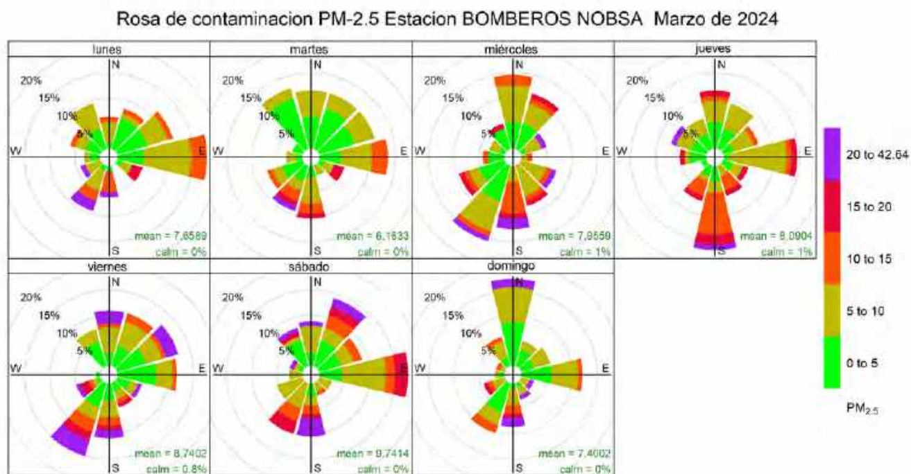
Figura 40. Rosa de contaminación PM-2.5 estación Bomberos Nobsa, marzo de 2024
