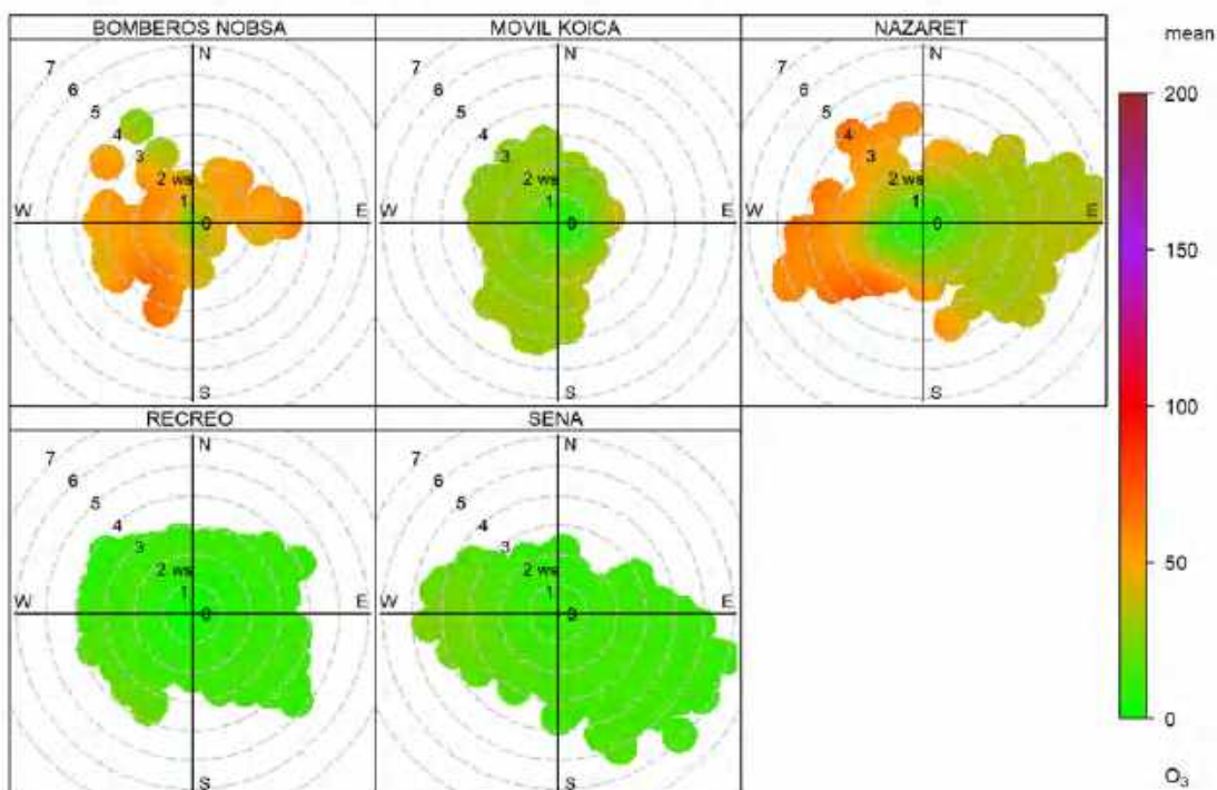
Figura 49. Gráfico Polar por estaciones O 3 , marzo de 2024 Grafica Polar O 3 Estaciones Marzo de 2024
