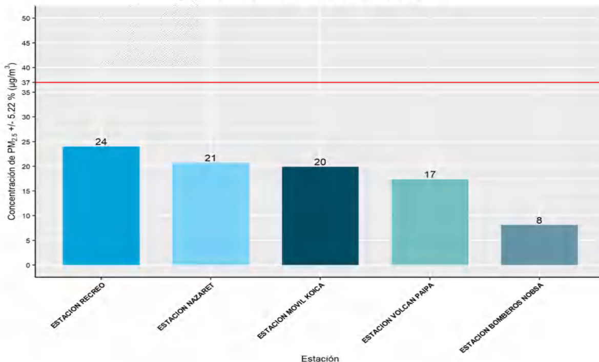
Figura 3. Promedio mensual PM-2.5 Red de monitoreo de calidad del aire CORPOBOYACA Concentración de PM 2.5 . MARZO de 2024
