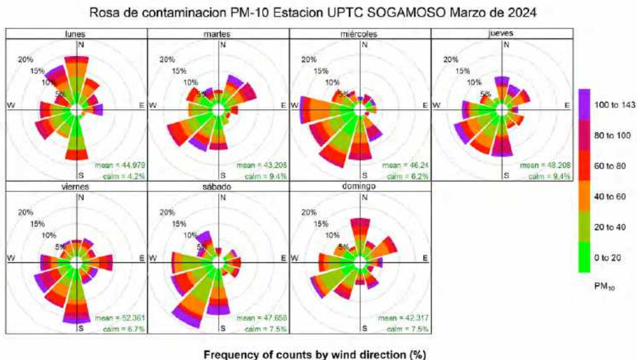
Figura 44. Rosa de contaminación PM-10 estación UPTC Sogamoso, marzo de 2024
