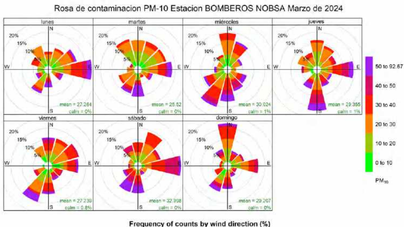
Figura 39. Rosa de contaminación PM-10 estación Bomberos Nobsa, marzo de 2024
