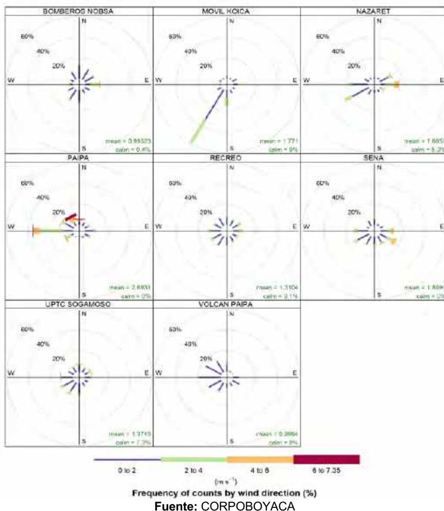
Figura 74. Velocidad y dirección del viento por estaciones marzo de 2024
