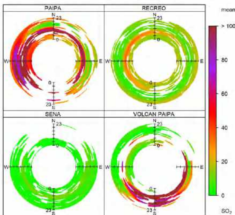
Figura 54. Gráfico anular SO 2 estaciones, marzo de 2024 Grafica anular SO 2 Estaciones Marzo de 2024
