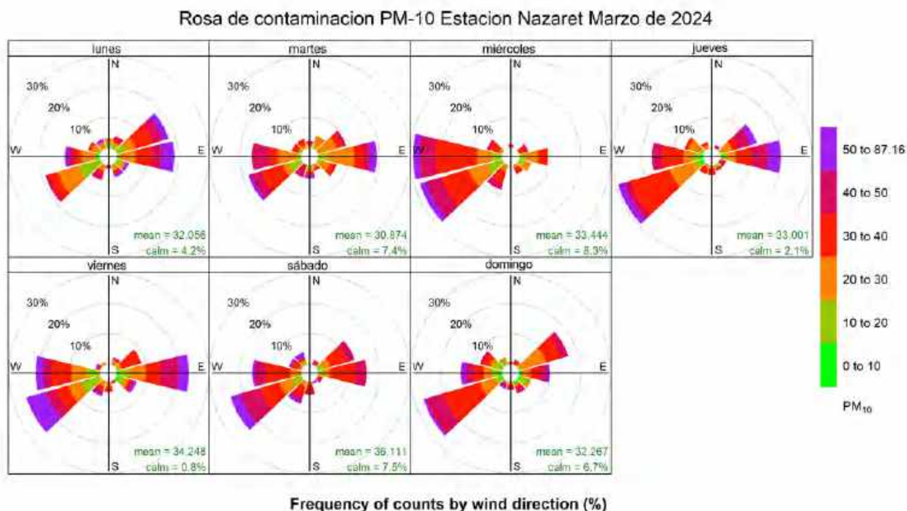
Figura 41. Rosa de contaminación PM-10 estación Nazaret, marzo de 2024
