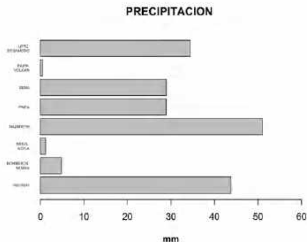
Figura 76. Precipitación registrada en las estaciones, marzo de 2024
