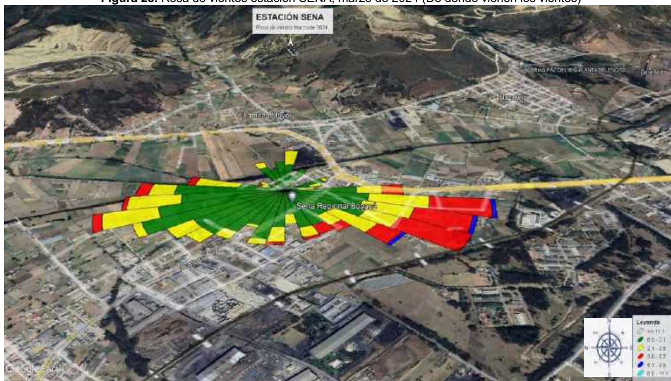
Figura 28. Rosa de vientos estación SENA, marzo de 2024 (De dónde vienen los vientos)
