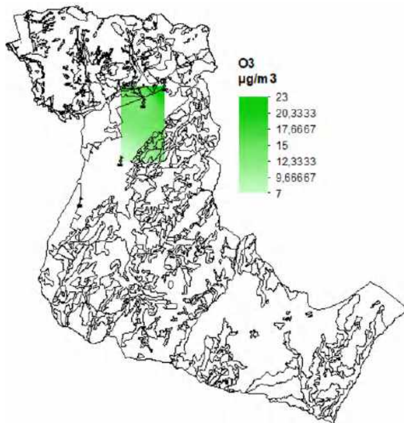
Figura 9. Promedio mensual O 3 Valle de Sogamoso
