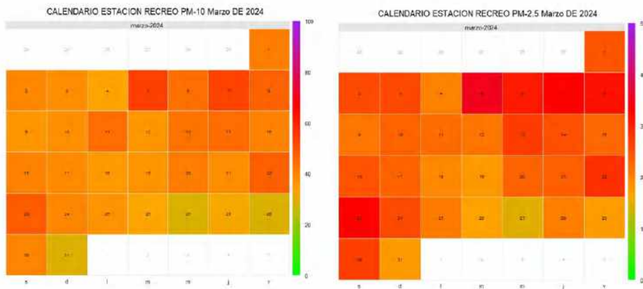
Figura 58. Calendario estación Recreo, marzo de 2024
