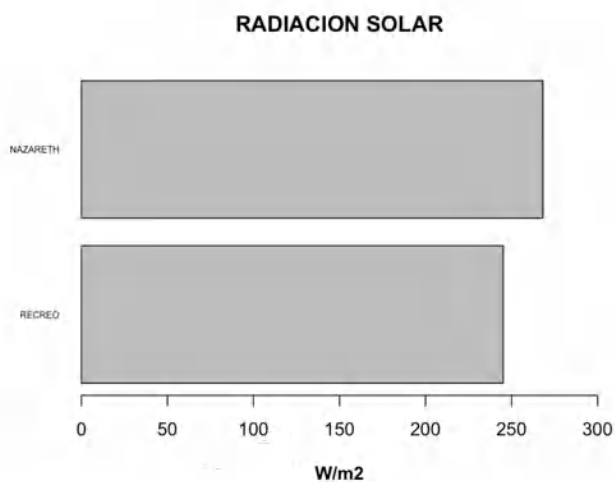
Figura 79. Radiación Solar registrada en estaciones, marzo de 2024
