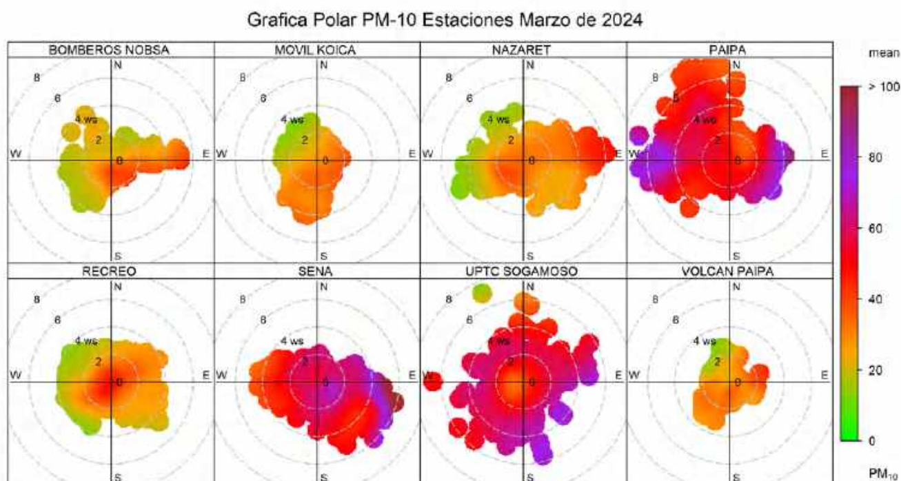
Figura 46. Gráfico polar por estaciones PM-10, marzo de 2024
