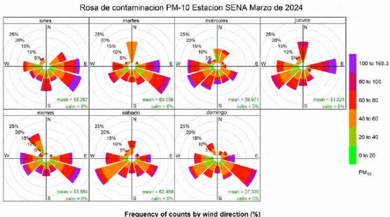
Figura 36. Rosa de contaminación PM-10 estación SENA, marzo de 2024
