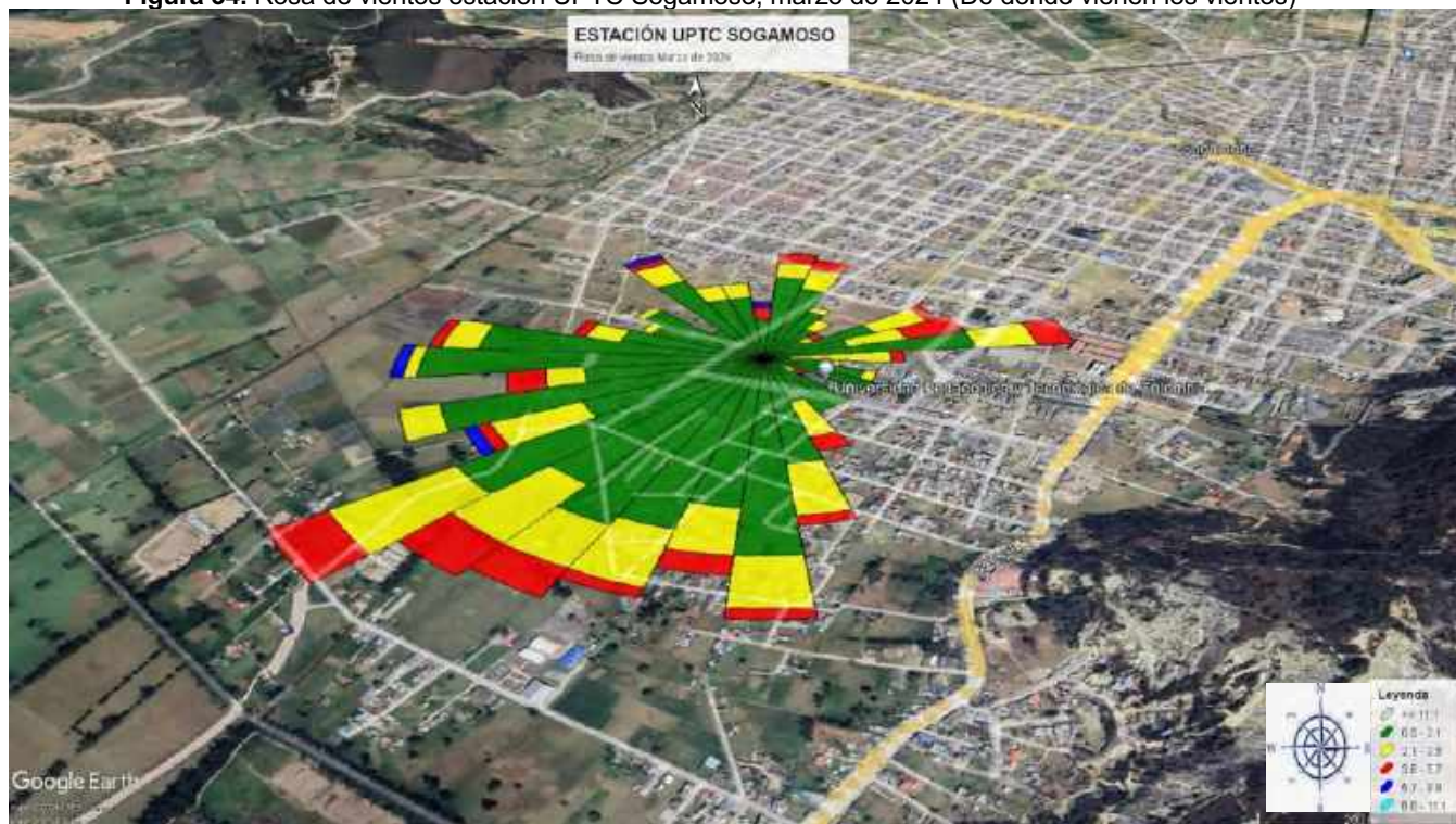
Figura 34. Rosa de vientos estación UPTC Sogamoso, marzo de 2024 (De dónde vienen los vientos)
