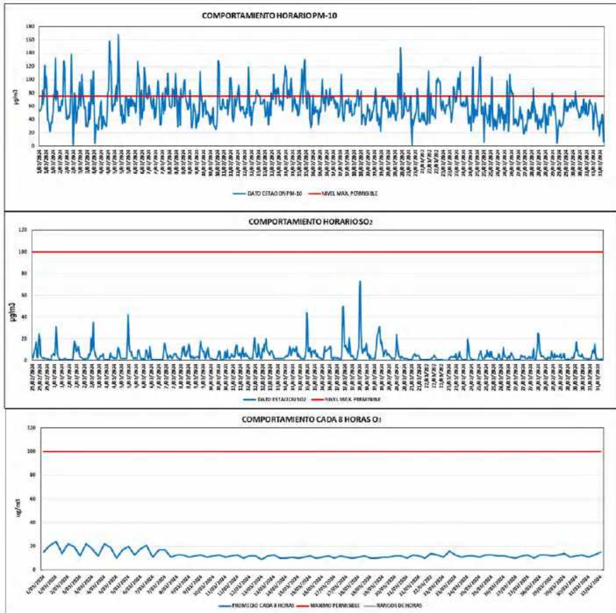
Figura 70. Comportamiento horario PM-10, SO 2 y O 3 , marzo de 2024
