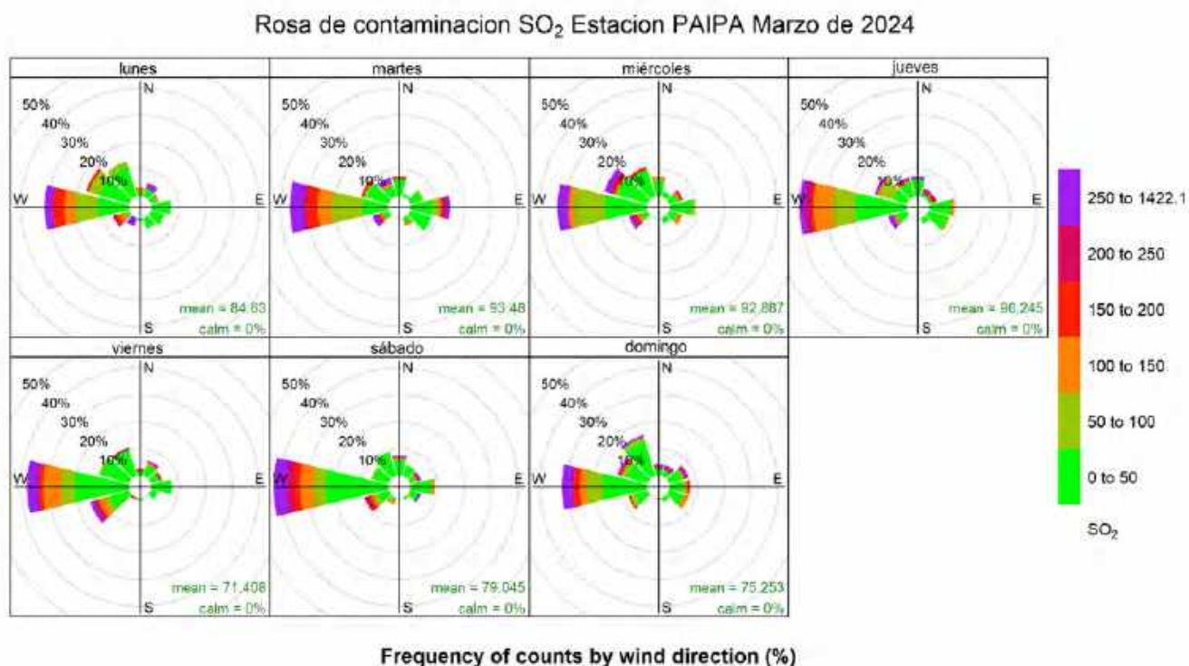
Figura 38. Rosa de contaminación SO 2 estación Paipa, marzo de 2024
