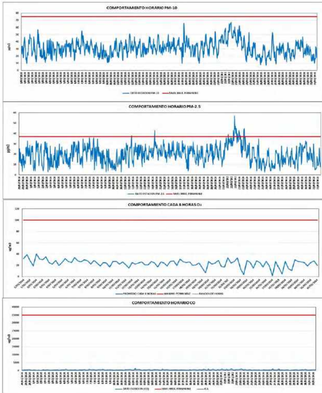
Figura 73. Comportamiento horario PM-10, PM-2.5, CO y O 3 marzo de 2024
