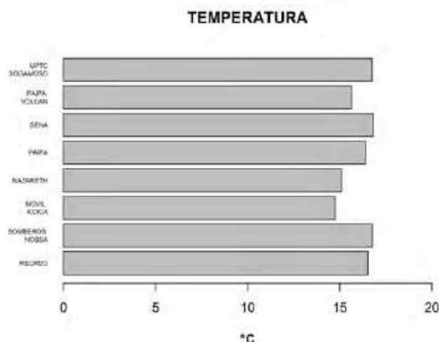
Figura 75. Temperatura registrada en estaciones, marzo de 2024
