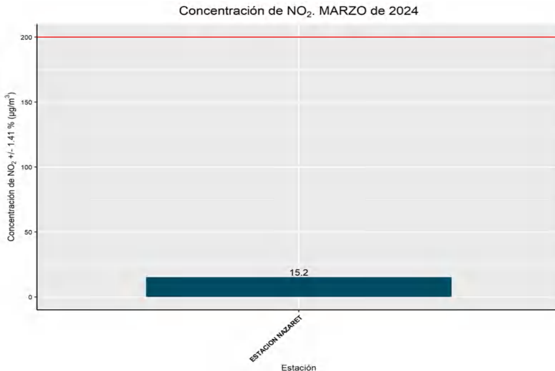
Figura 7. Promedio mensual NO 2 Red de monitoreo de calidad del aire CORPOBOYACA
