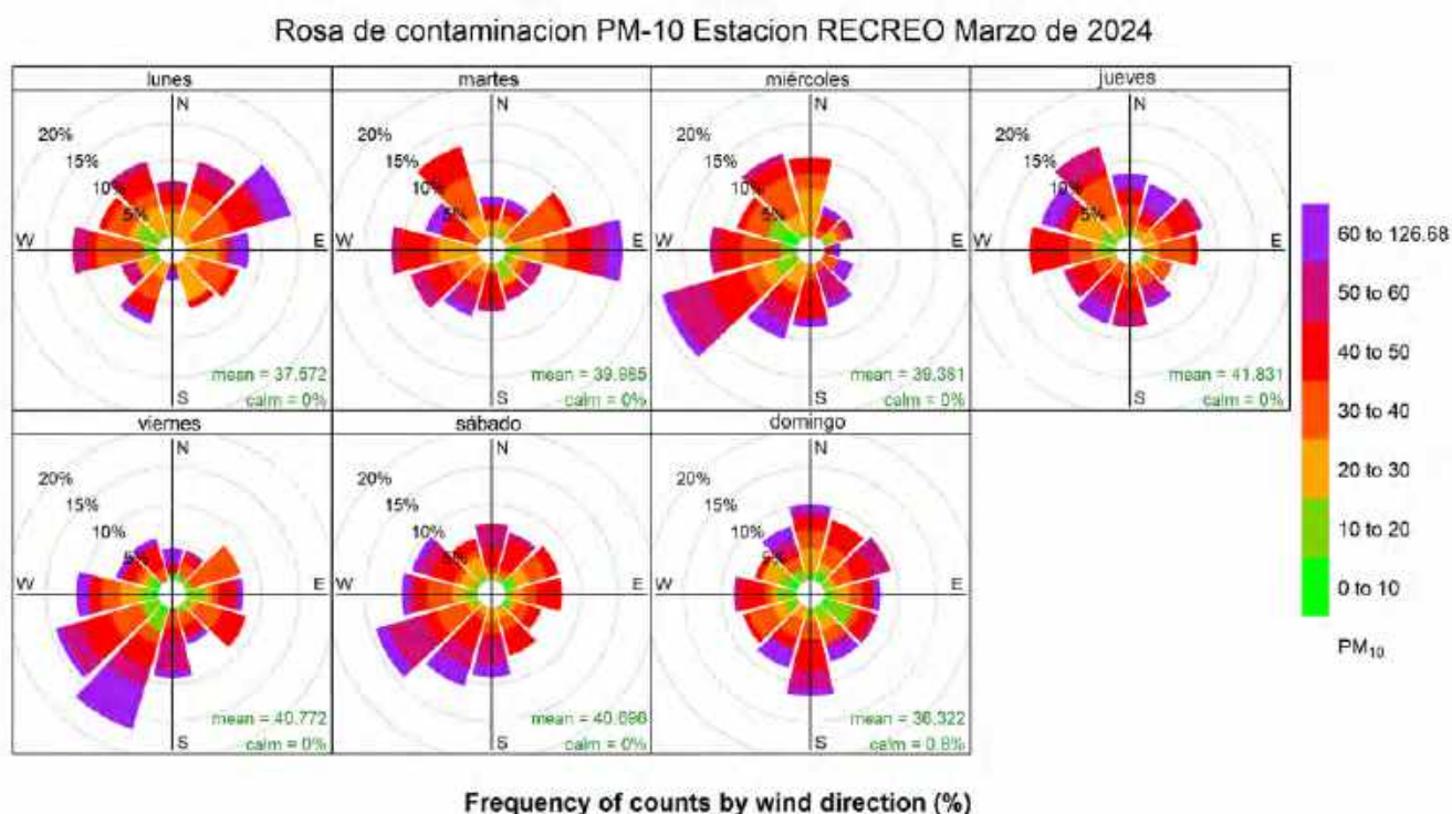
Figura 35. Rosa de contaminación PM-10 estación Recreo, marzo de 2024
