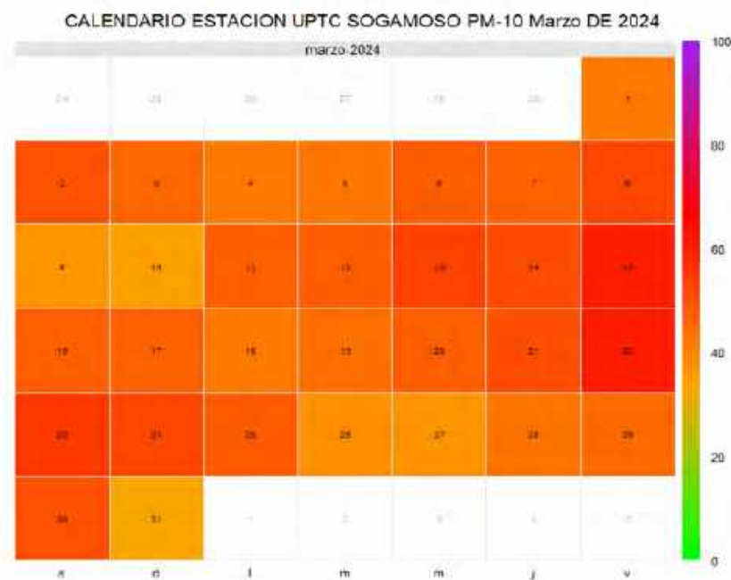
Figura 65. Calendario estación UPTC Sogamoso, marzo de 2024
