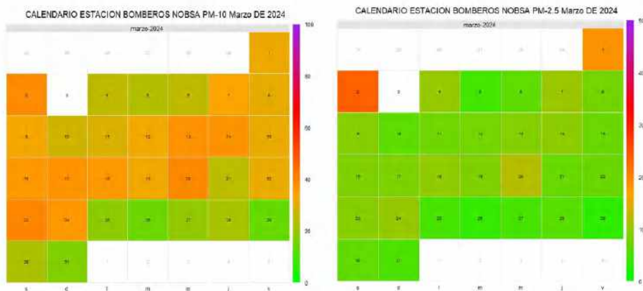
Figura 62. Calendario estación Bomberos Nobsa, marzo de 2024
