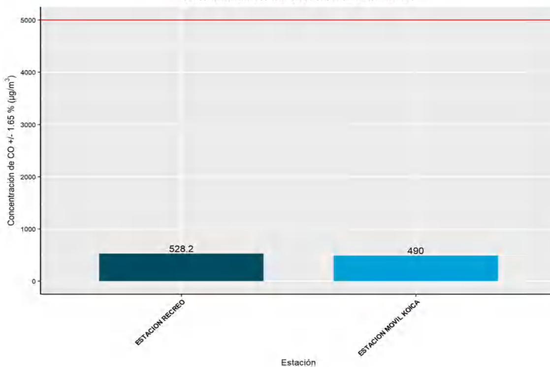
Figura 10. Promedio mensual CO Red de monitoreo de calidad del aire CORPOBOYACA Concentración de CO. MARZO de 2024
