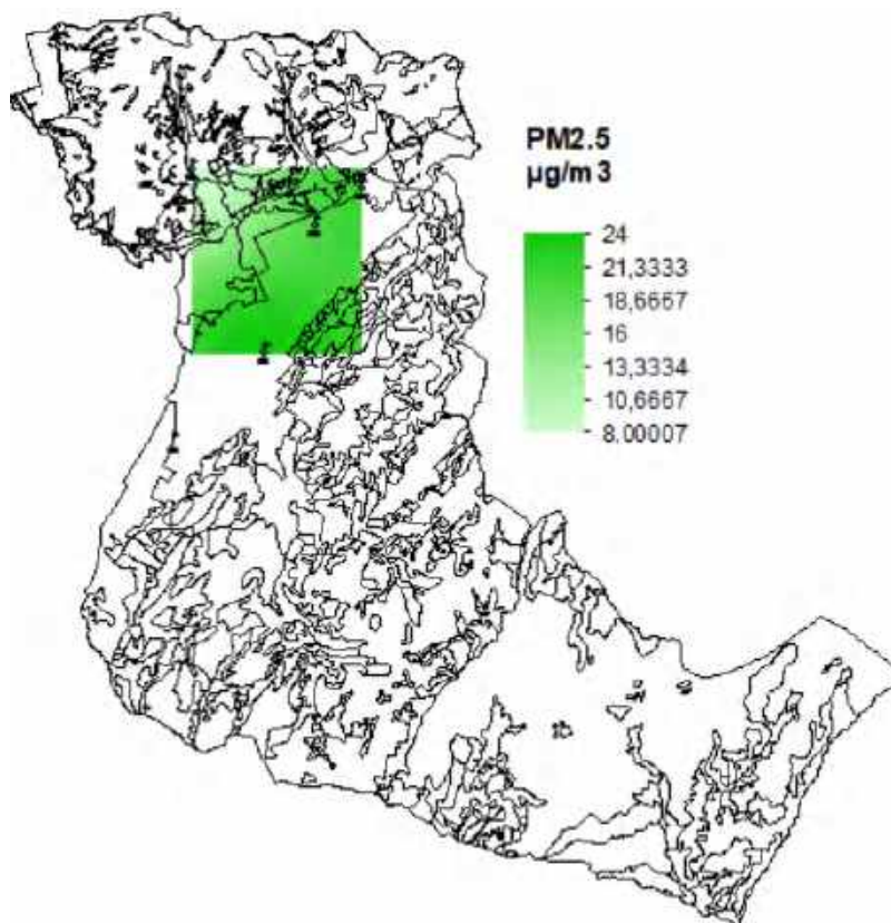
Figura 4. Promedio mensual PM-2.5 Valle de Sogamoso
